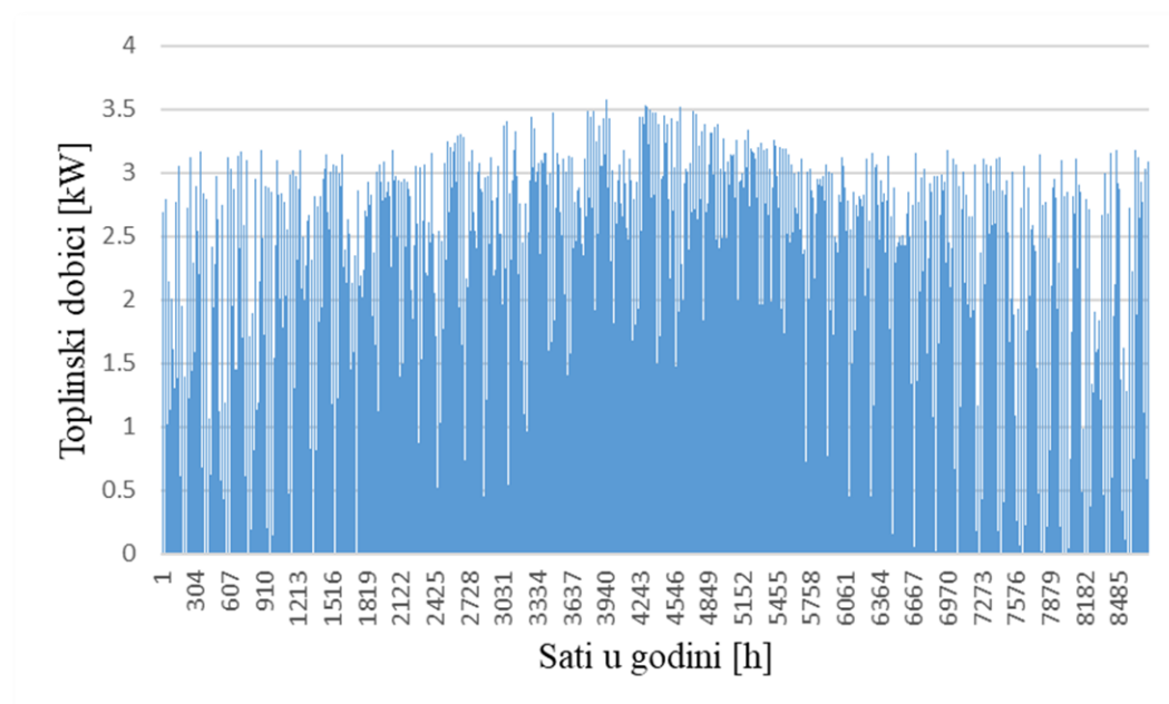
Slika 12 Solarni toplinski dobici
