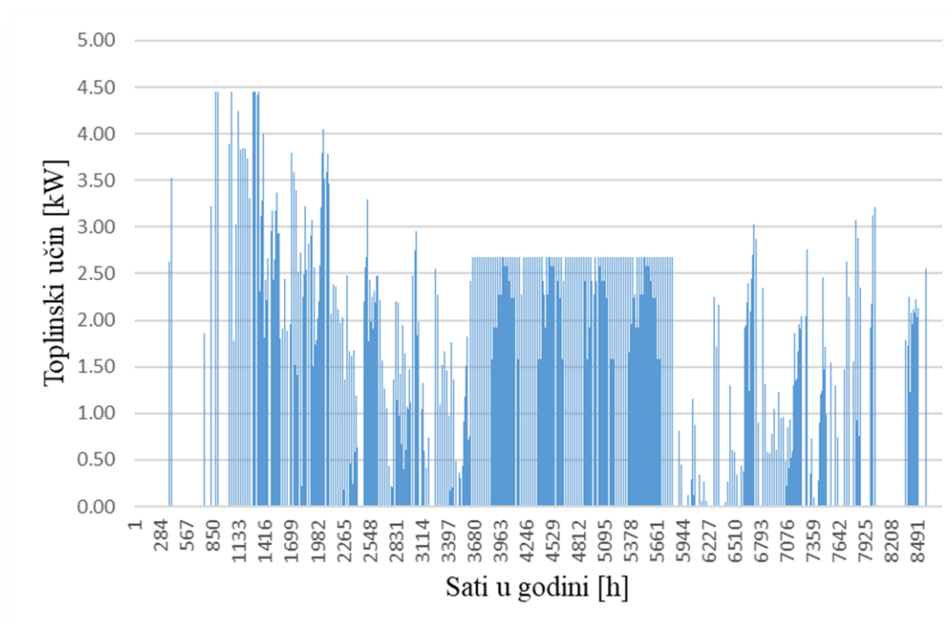
Slika 48 Pokrivanje potreba grijanja i PTV-a električnom energijom preko dizalice topline scenarija B
