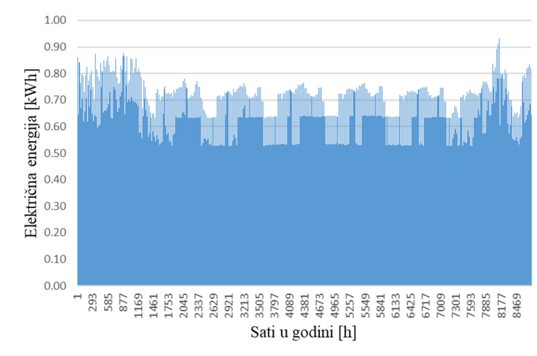
Slika 25 Utrošak električne energije dizalice topline i električnog grijača za zagrijavanje PTV-a Godišnja potrebna količina električne energije dizalice topline za zagrijavanje PTV-a iznosi 3061,75 kWh.
