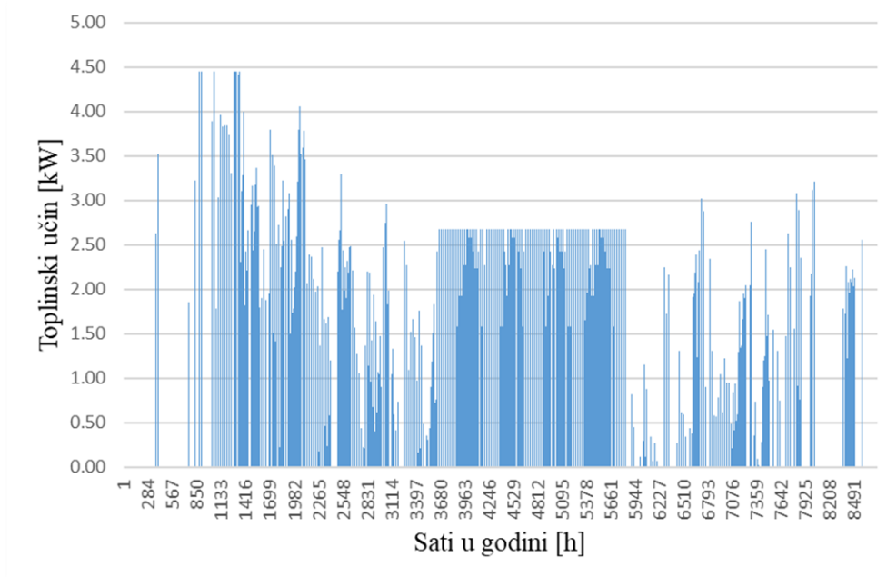
Slika 43 Pokrivanje potreba grijanja i PTV-a neiskorištenom proizvedenom električnom energijom preko dizalice topline
