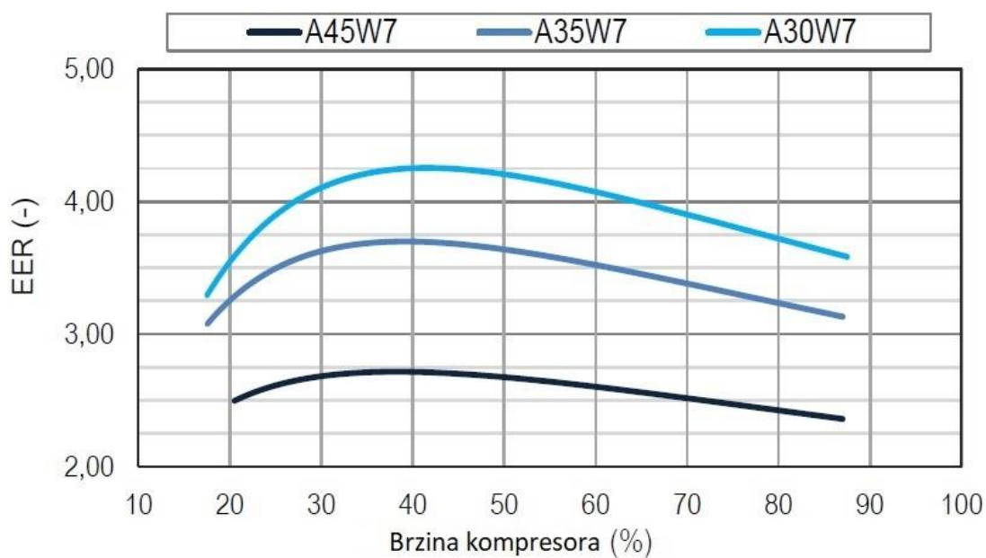
Slika 18 Ovisnost faktora hlađenja dizalice topline s obzirom na parcijalno opterećenje i temperaturu vanjskog zraka dobiveno od proizvođača odabrane dizalice topline [24]
