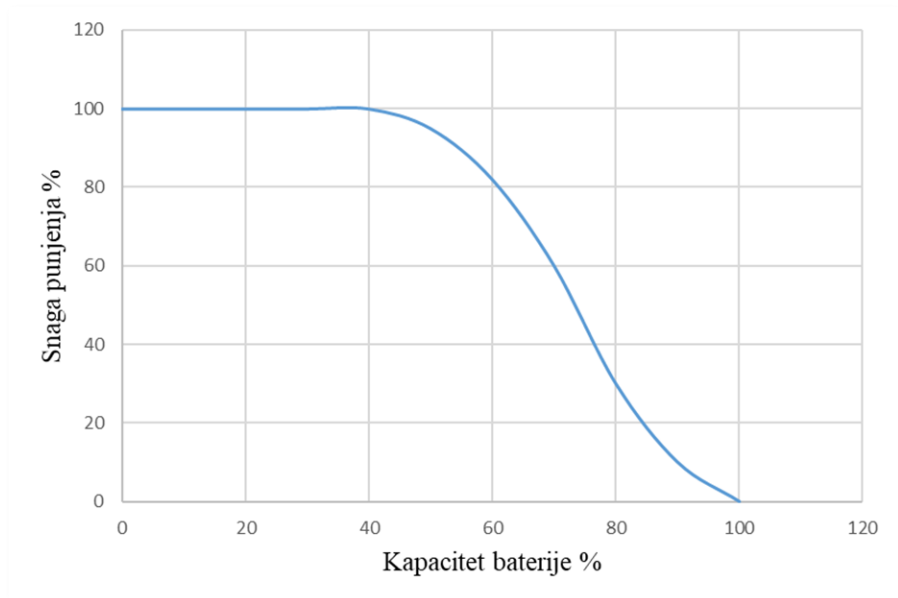
Slika 37 Ovisnost kapaciteta baterije i snage punjenja
