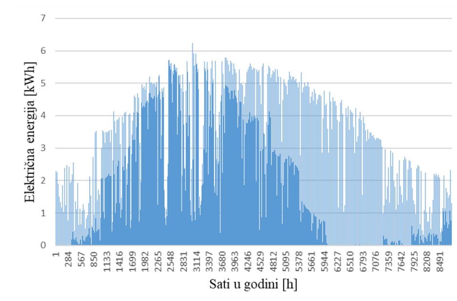
Slika 31 Proizvodnja električne energije iz solarne elektrane
