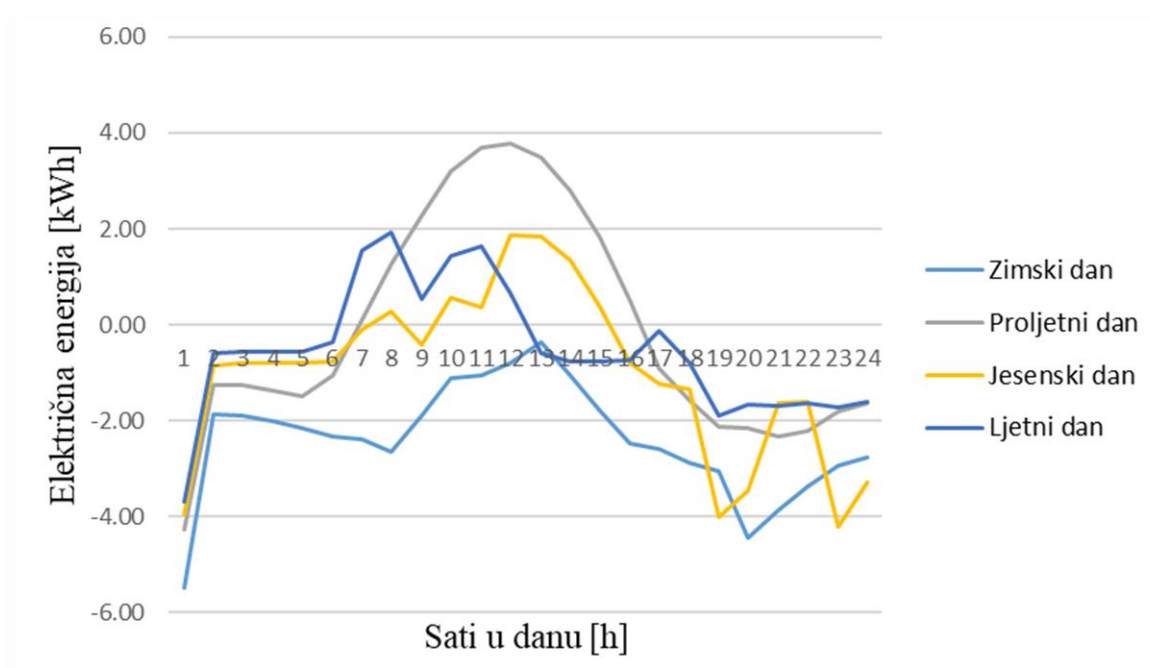
Slika 41 Preuzeta i predana električna energija u mrežu po karakterističnim danima u godini
