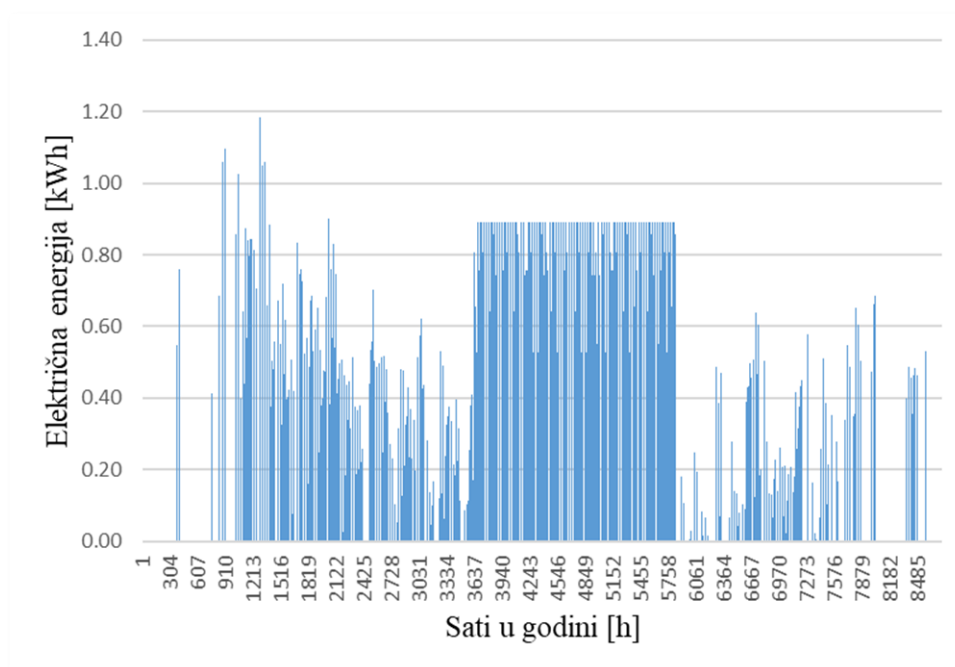
Slika 44 Ušteda električne energije na dizalici topline
