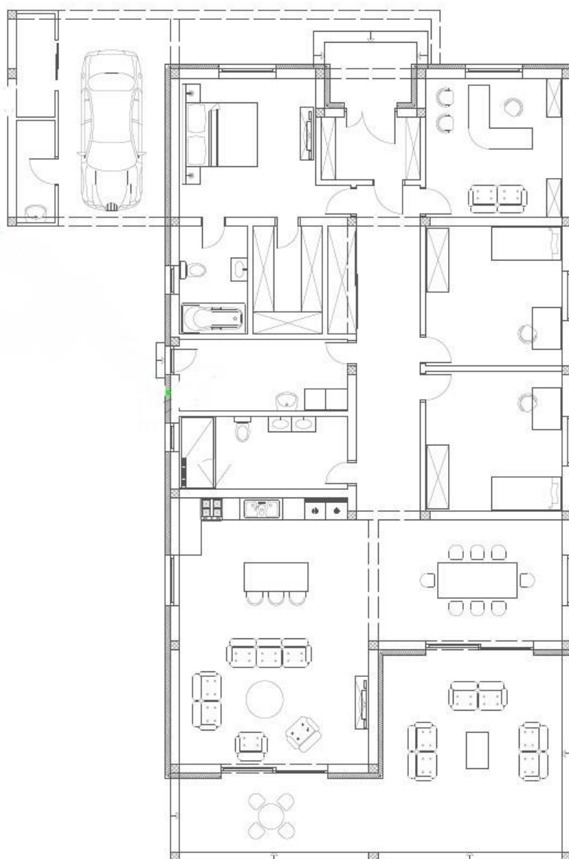
Slika 5 Tlocrt prizemlja [3]
