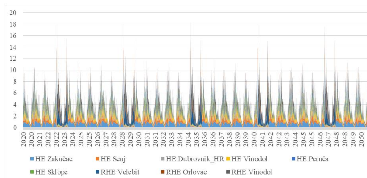
Dodatak 4. Satni dotoci akumulacijskih hidroelektrana u scenariju bez utjecaja klimatskih promjena
