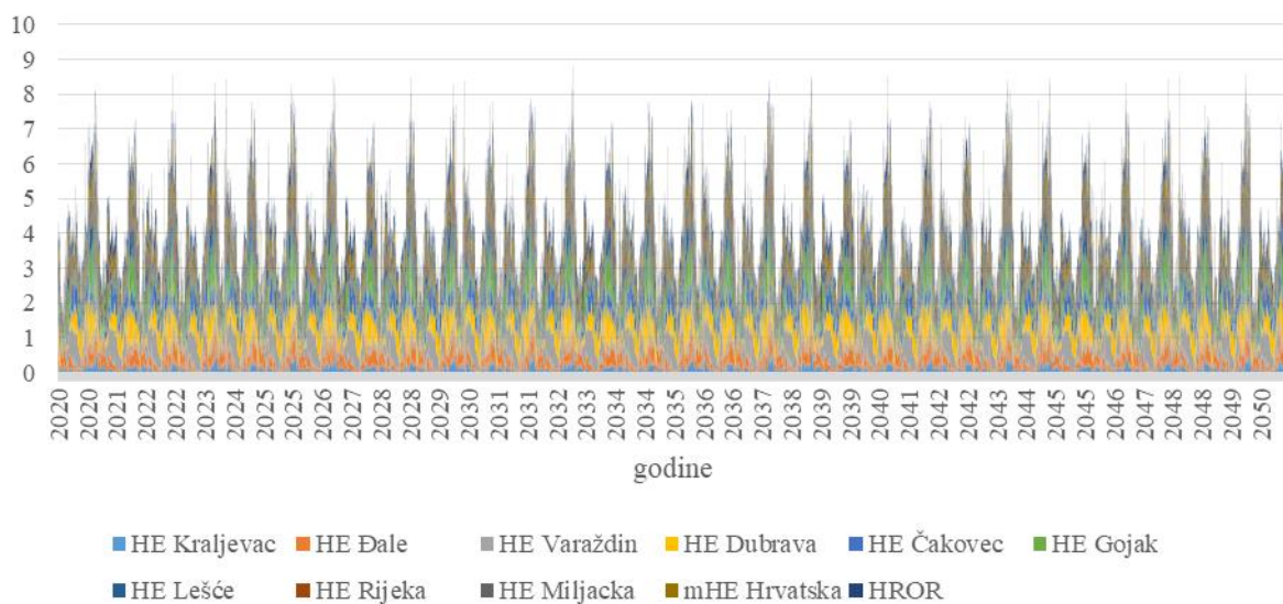
Dodatak 5. Satni faktori opterećenja protočnih hidroelektrana u scenariju očekivanog razvoja
