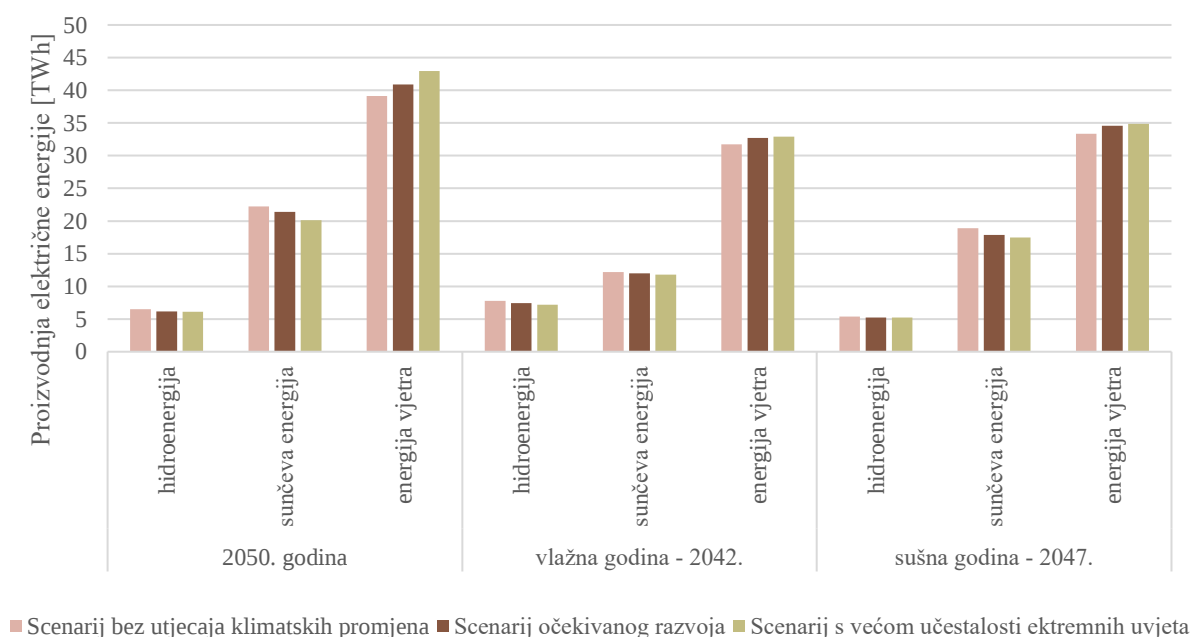
Slika 84. Usporedba proizvodnje po scenarijima iz fotonaponskih i vjetroelektrana za 2050., karakterističnu sušnu i vlažnu godinu
