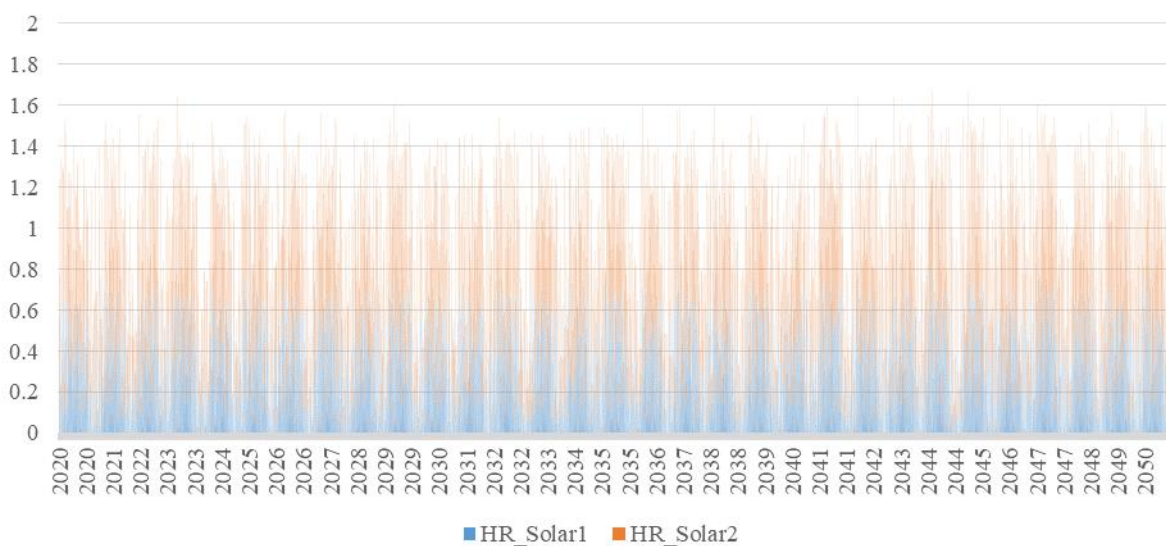
Dodatak 6. Satni faktori opterećenja fotonaponskih elektrana u scenariju očekivanog razvoja
