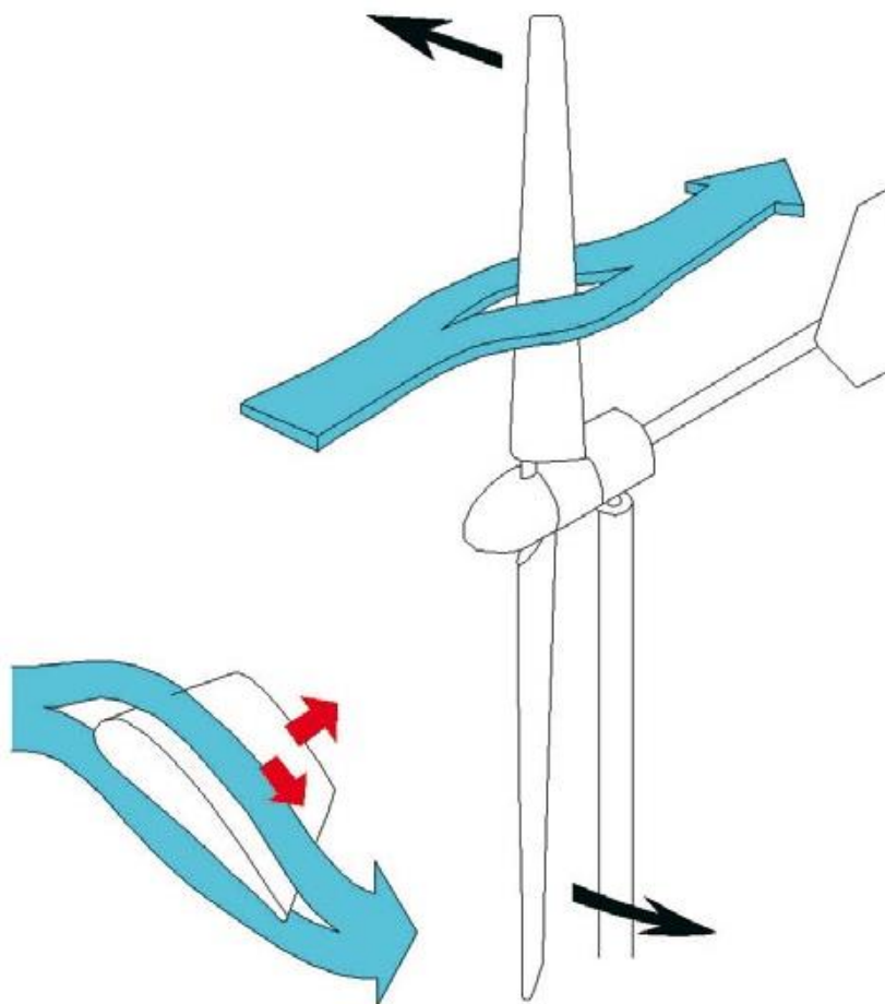
Slika 6. Sile uzgona – F_u i otpora - F_o na profile lopatica vjetroagregata [17]
