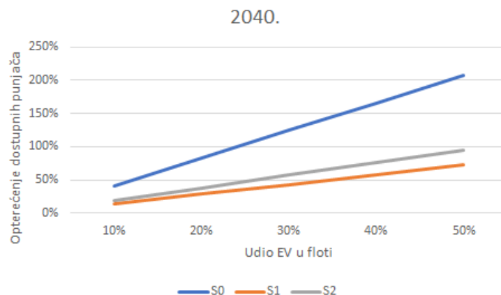
Slika 53. Ovisnost opterećenja dostupnih sporih punjača o udjelu EV u floti za 2040. godinu u zelenom području
