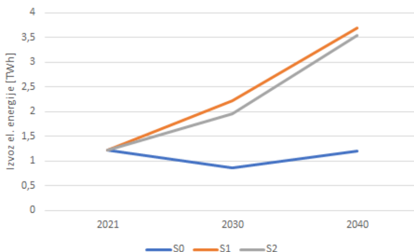
Slika 38. Izvoz električne energije za pojedini scenarij kroz godine
