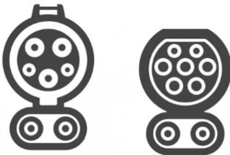
Slika 10. Priključak-TIP 3 [15]
