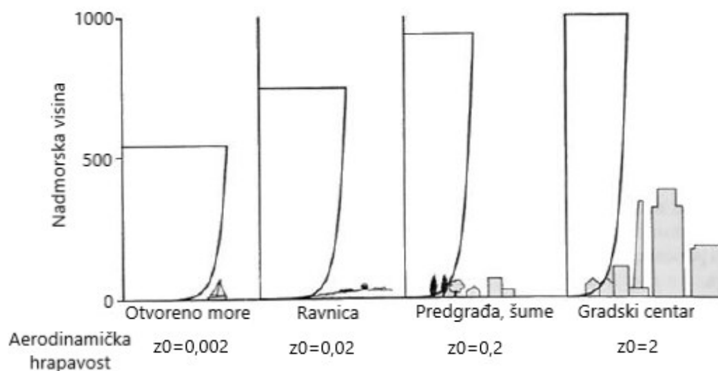
Slika 7.2: Aerodinamička duljina hrapavosti na raznim terenima [24]
