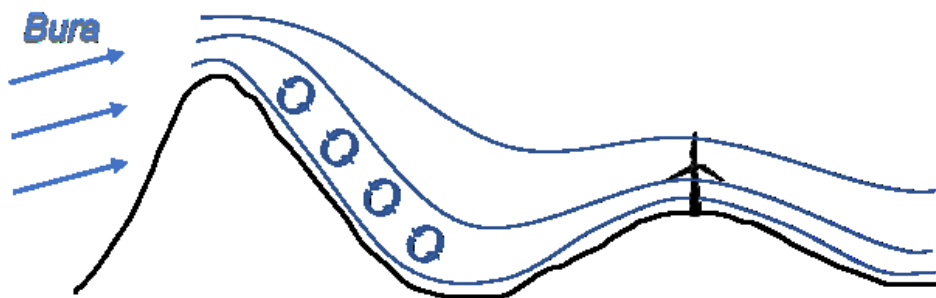
Slika 7.4: Pravilan položaj vjetroturbine iza planinskog masiva
