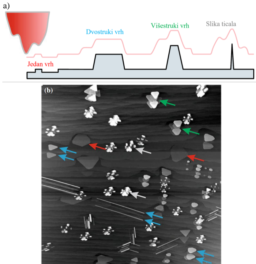
Slika 2.13. Mjerenje dvostrukim i višestrukim vrhom ticala [98] a) prikaz putanje dvostrukog i višestrukog vrha ticala, b) prikaz različitih značajki kao rezultat duplog i višestrukog ticala
