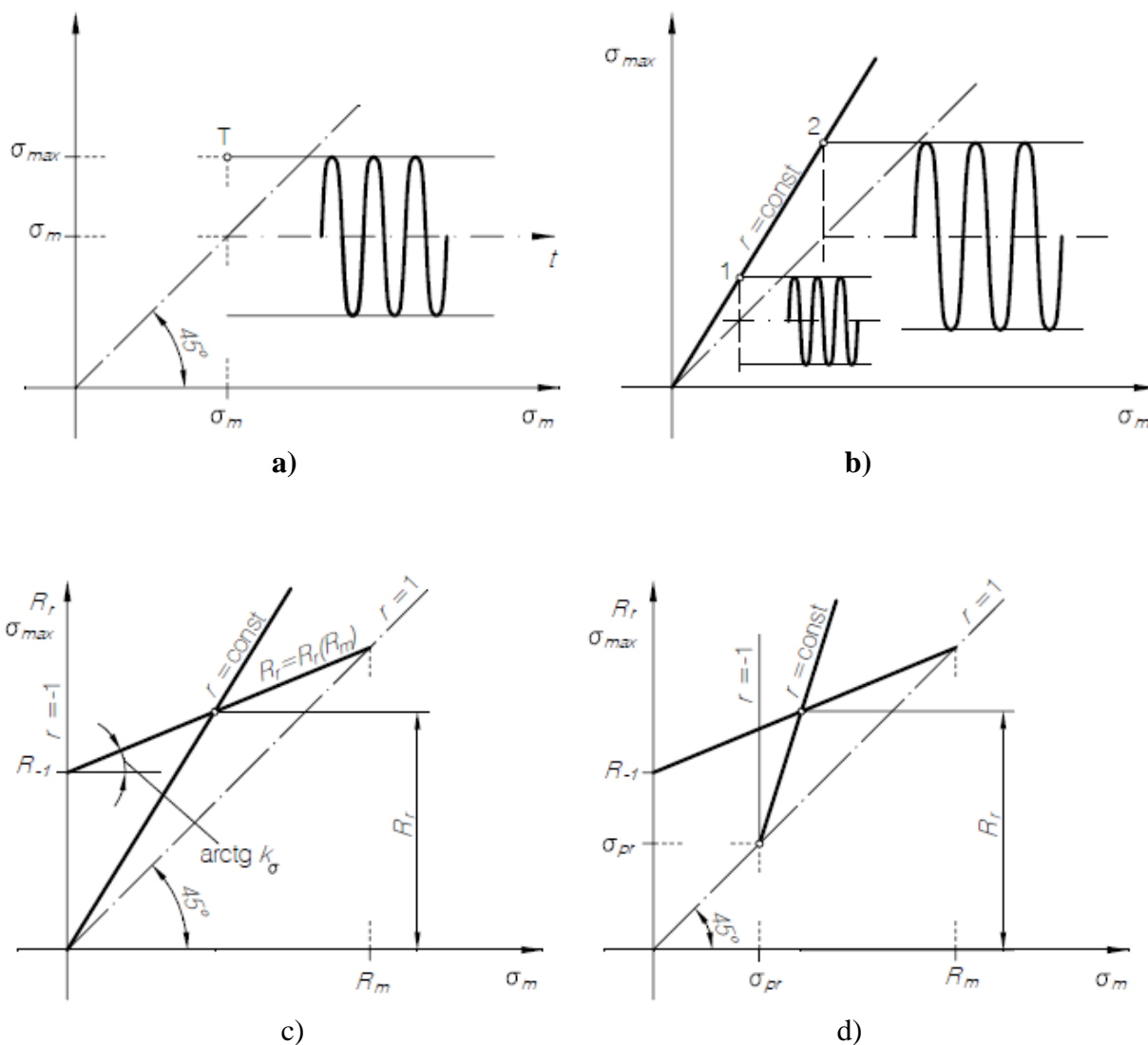
Slika 4.4 : Osnovni principi Smithovog dijagrama
