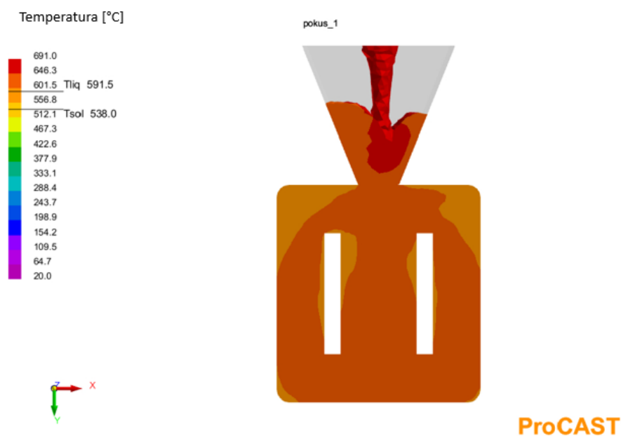
Slika 26. Ispunjenje kalupne šupljine i punjenje uljavnog sustava
