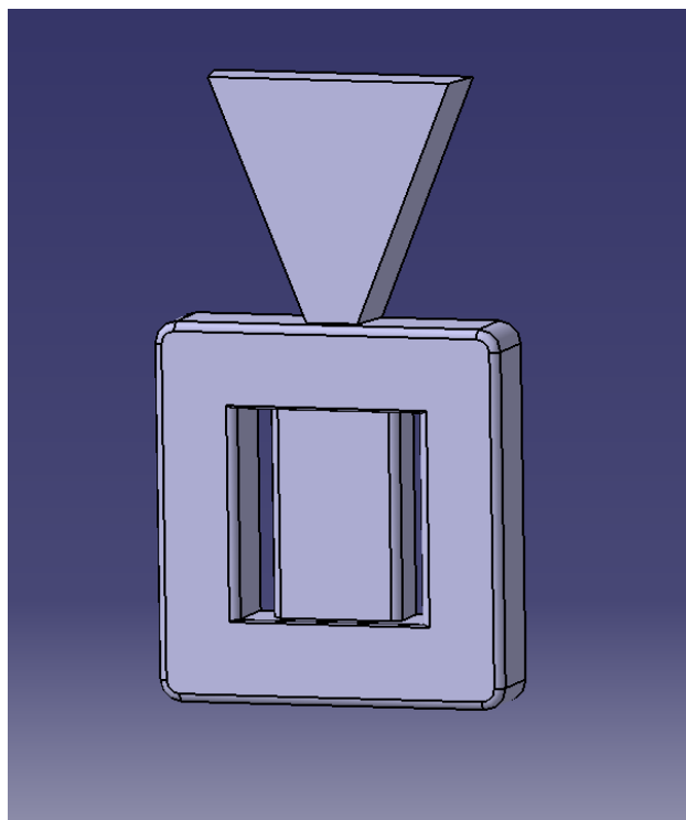
Slika 16. 3D model odljevka od aluminijske legure
