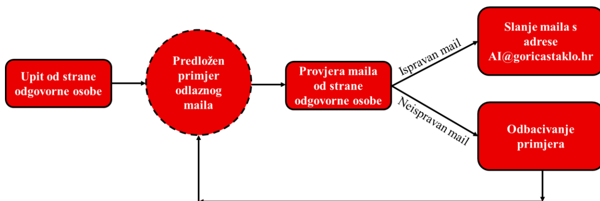
Slika 27. Shema funkcioniranja Agent E-mail
