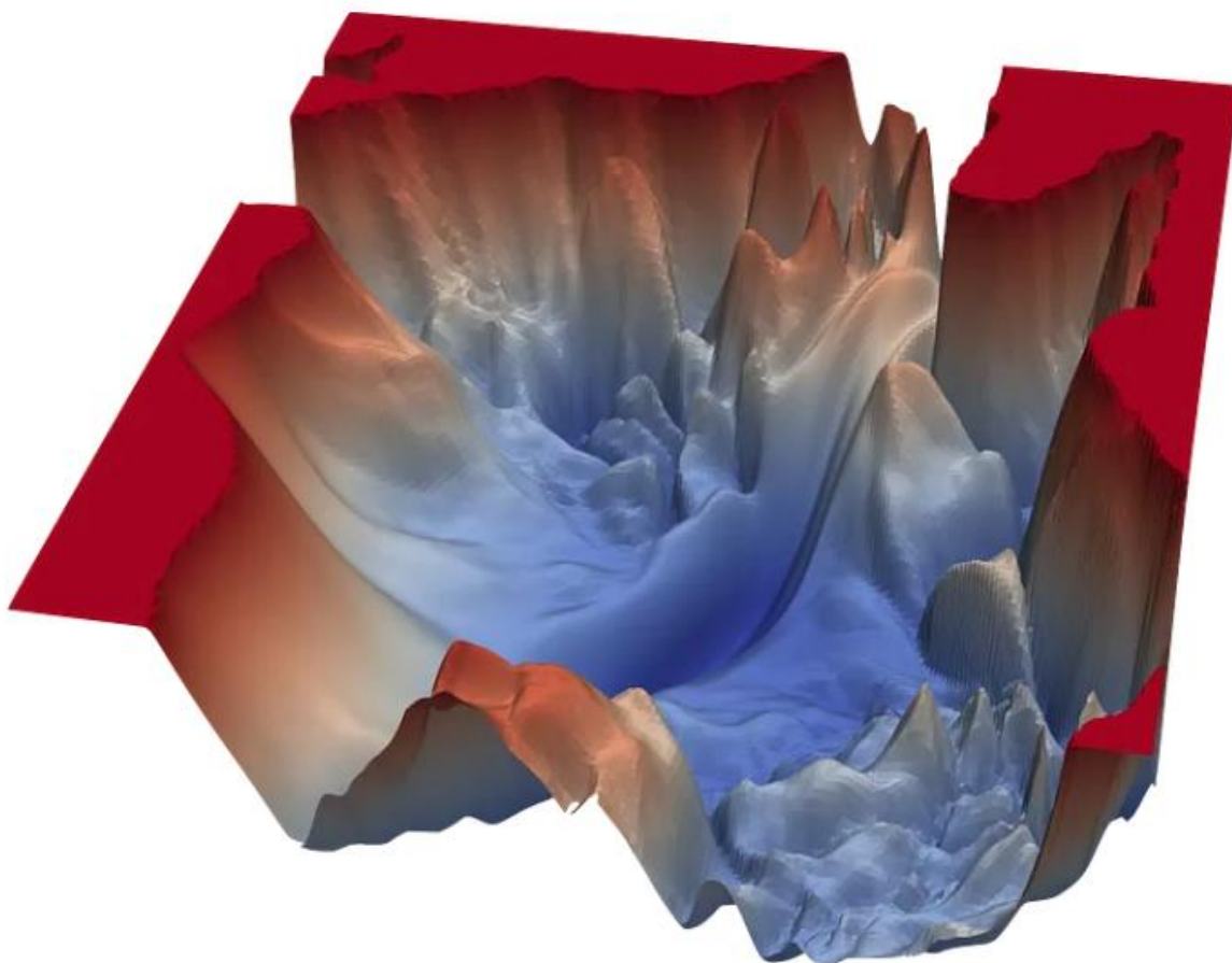
Slika 11. Krajoblik pogreške [32]
