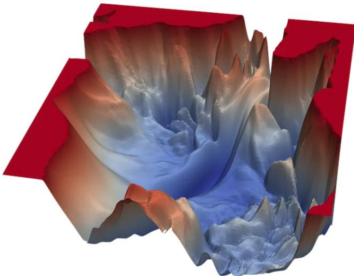
Slika 11. Krajoblik pogreške [32]
