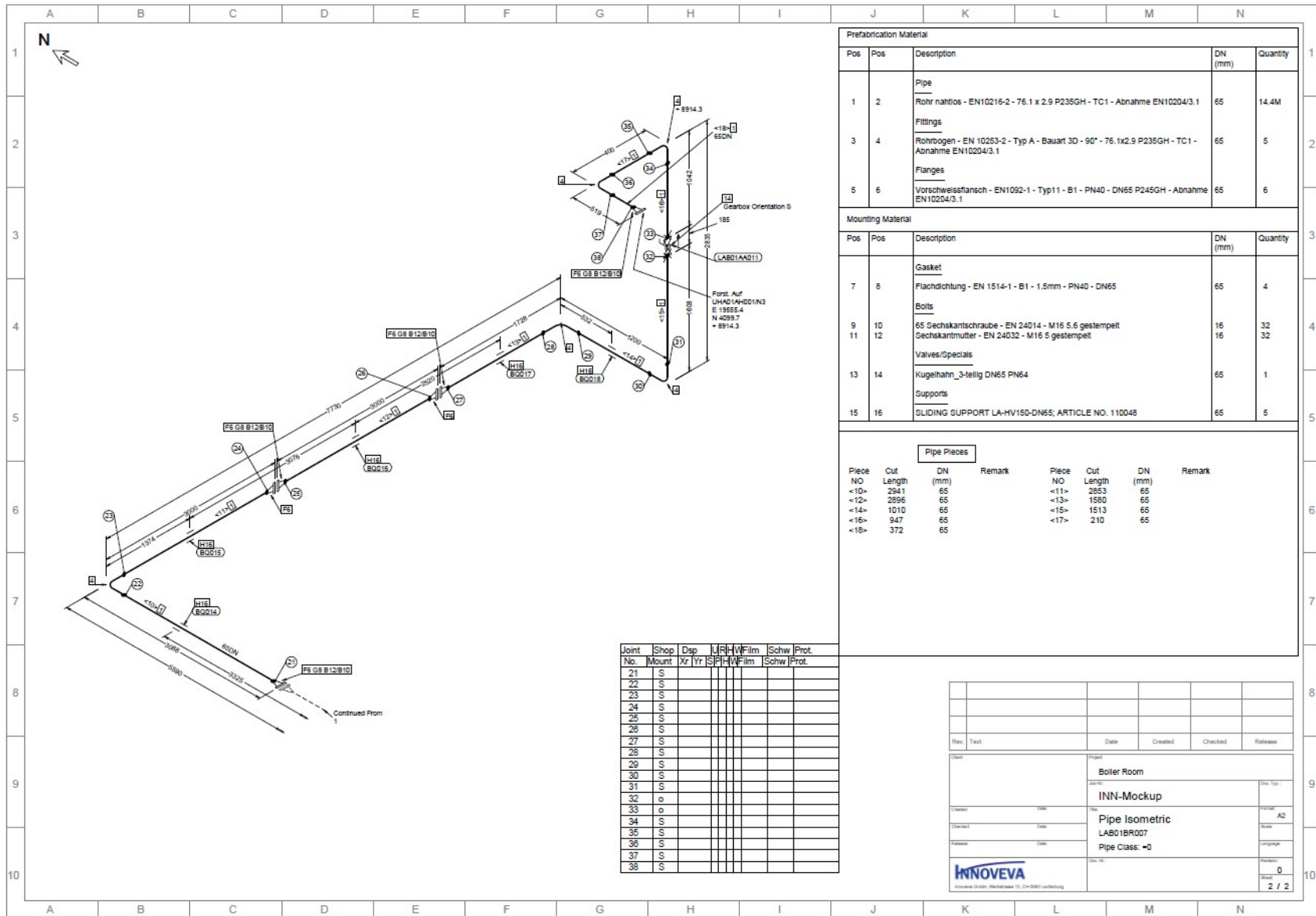
Slika 45. Cijevna izometrija 2/2
