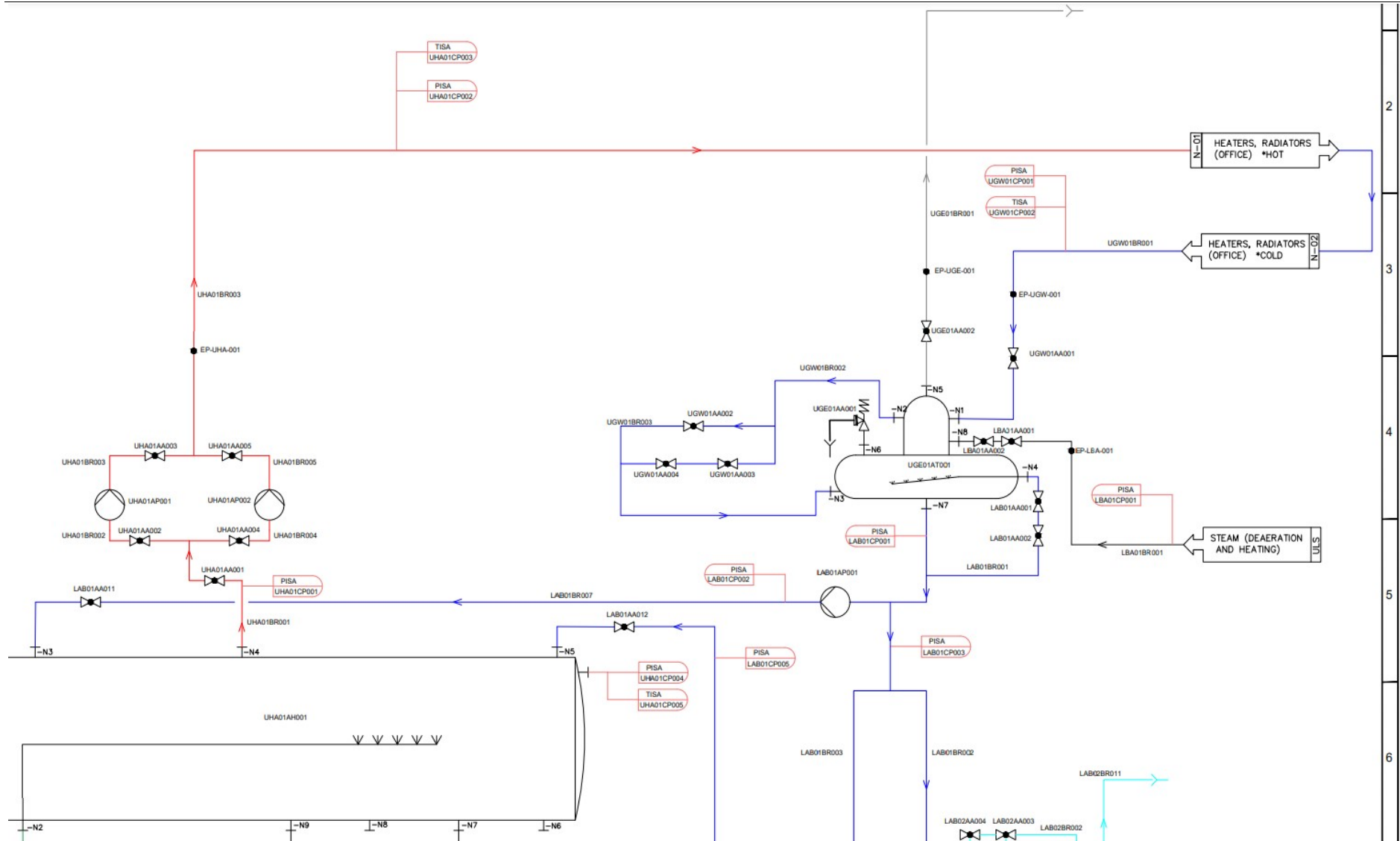
Slika 16. 2707-INN-DE-PID-001 – 2. dio
