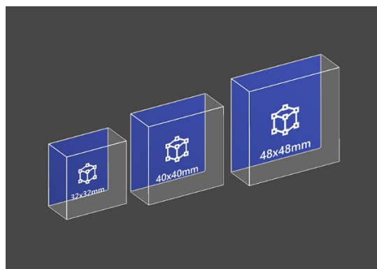
Slika 40. PressableButtonHoloLens2 gumb
