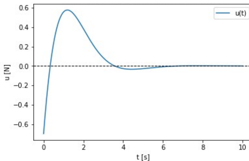
Slika 5.2 Vremenska ovisnost upravljačke varijable
