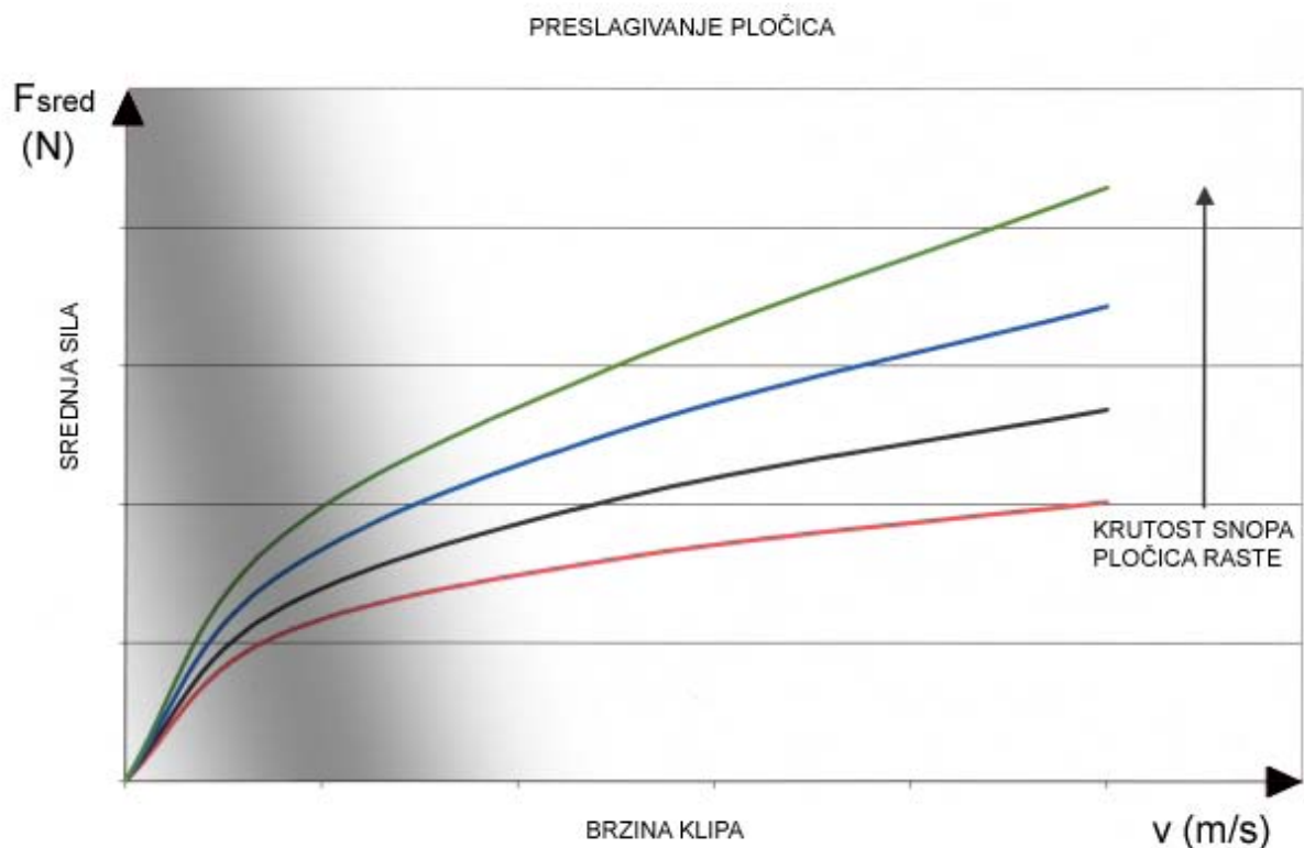
Slika 3.2 Preslagivanje pločica
