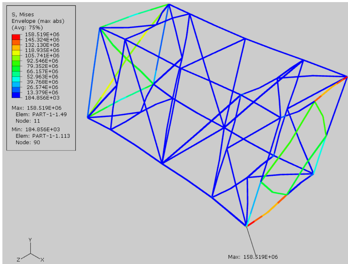
Slika 4.10 Rekonstruirana rešetka - prikaz maksimalnih ekvivalentnih naprezanja – djelovanje horizontalne vlačne sile F=150 kN
