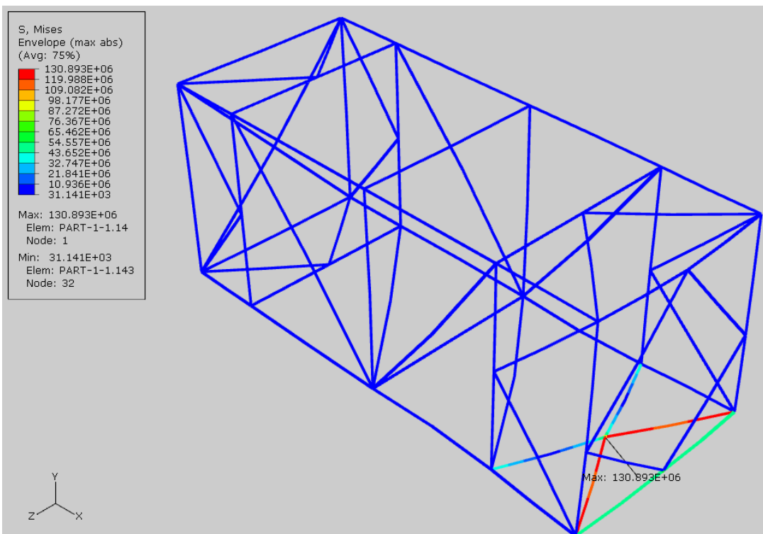
Slika 4.14 Rekonstruirana rešetka - prikaz maksimalnih ekvivalentnih napreznja – djelovanje uzdužne inercijske sile na podnu rešetku I
