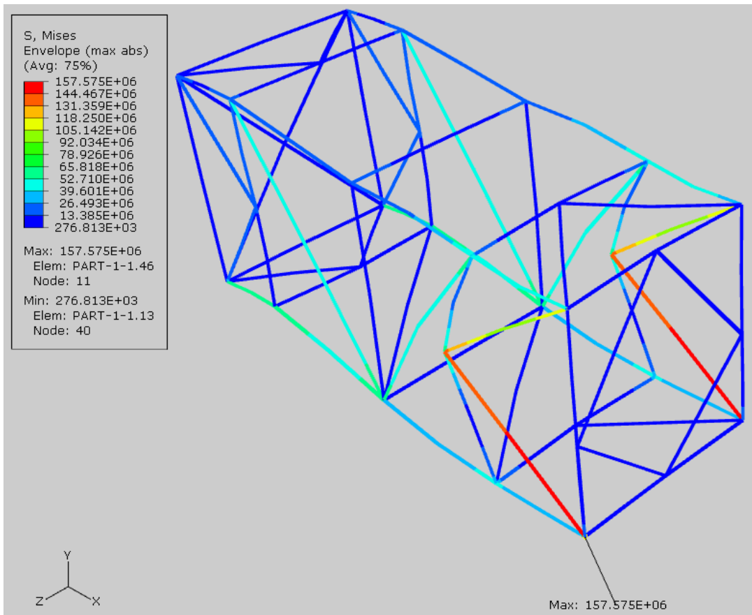
Slika 4.13 Rekonstruirana rešetka - prikaz maksimalnih ekvivalentnih napreznja – djelovanje uzdužne inercijske sile na bočne rešetke II
