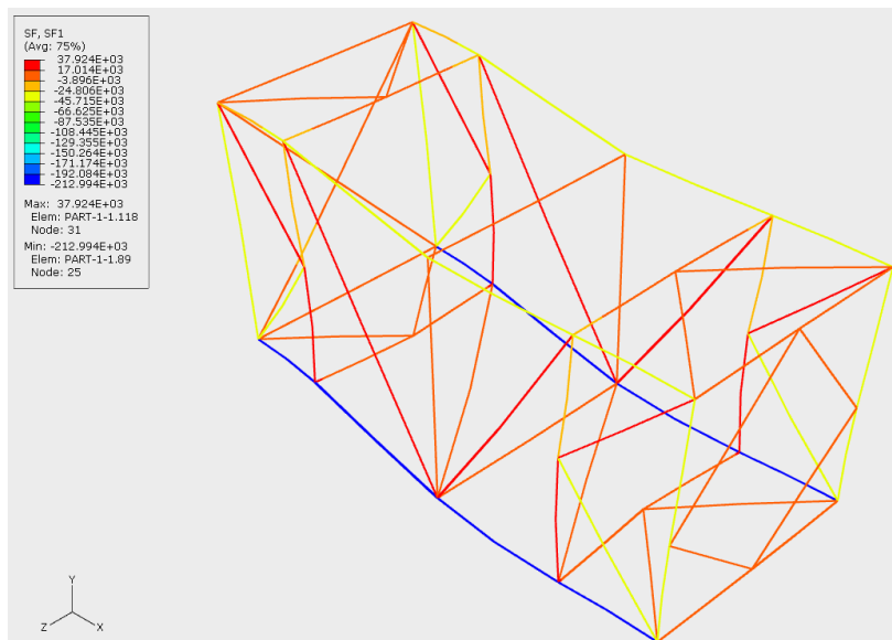
Slika 3.12 Raspodjela osnovih sila izražena u njutnima [N]
