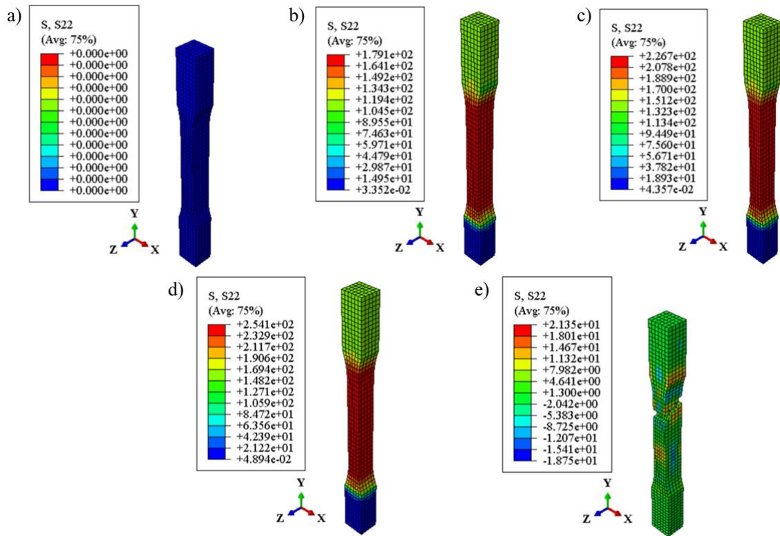
Slika 5.11. Vremenski tok simulacije - 6,5 g/cm 3 : a) 0,0 sekundi, b) 5,25 sekundi, c) 10,5 sekundi, d) 15,75 sekundi, e) 21,0 sekundi
