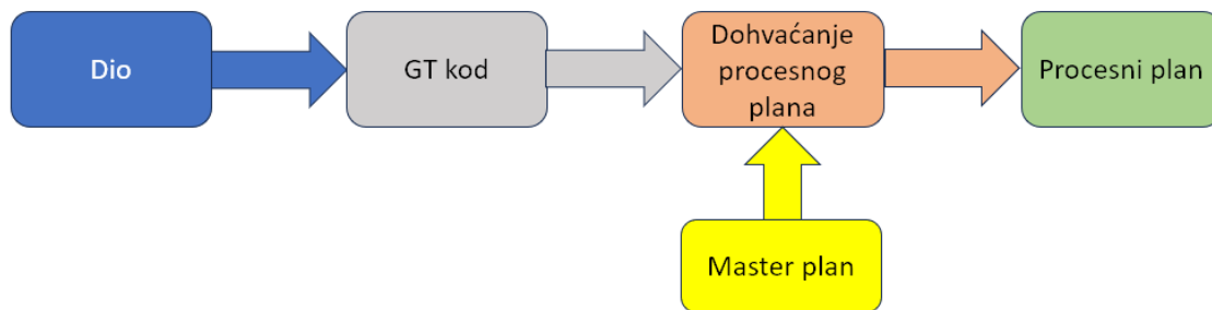
Slika 3. Generativni pristup [5]
