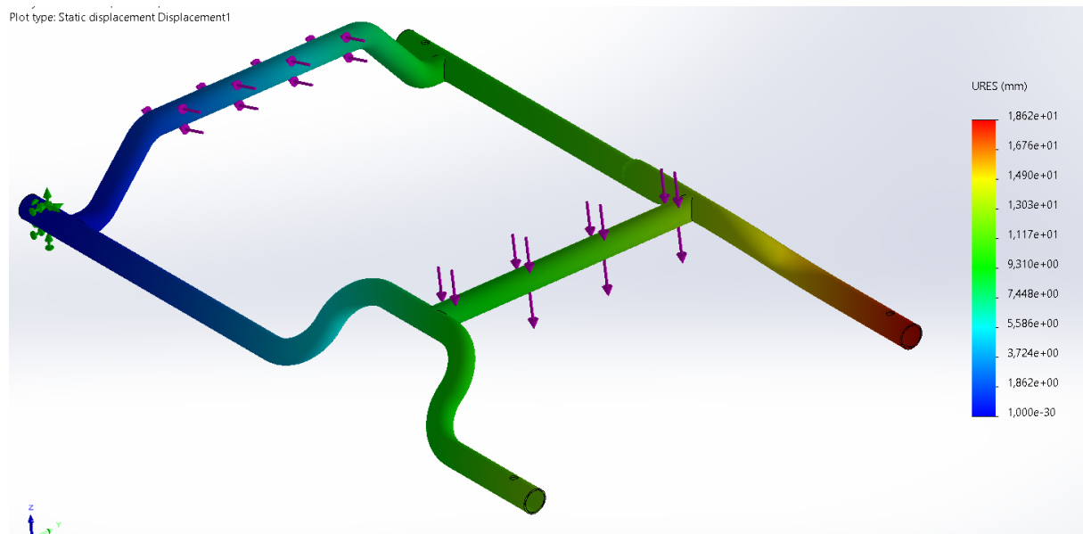
Slika 44. Rezultati pomaka pri zakočenom stražnjem kotačiću
