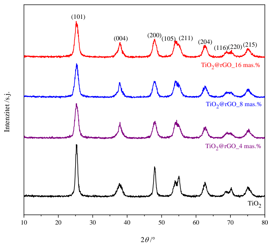
Slika 4.7. Difraktogrami uzoraka nanočestica \text{TiO}_2 i \text{TiO}_2@\text{rGO} nanokompozita.
