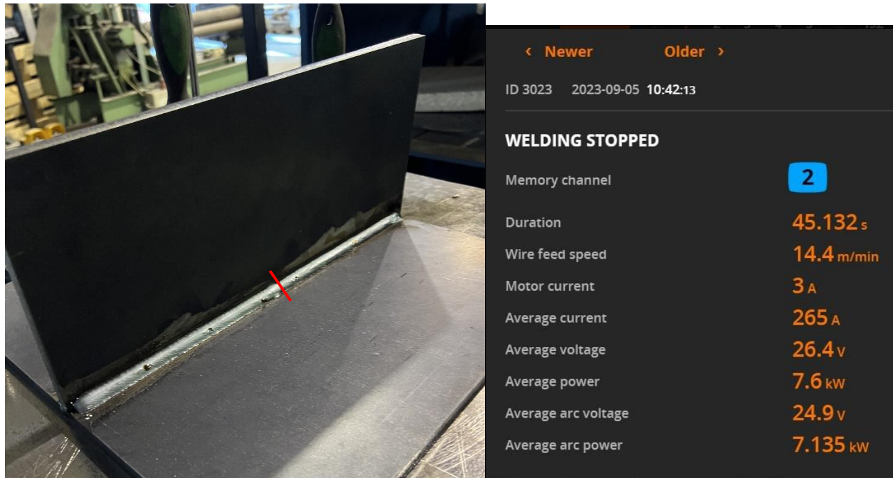
Slika 37. Prikaz drugog zavara s naznačenim trenutkom promjene zavara i parametri zavarivanja
