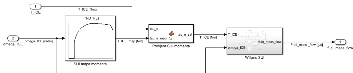
Slika 43. Simulink model motora s unutarnjim izgaranjem.
