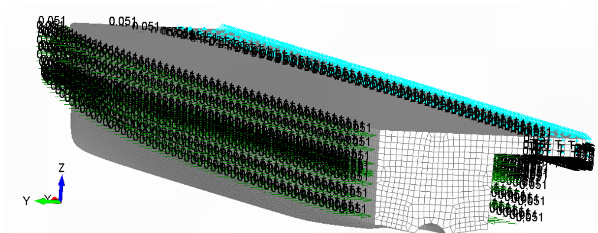
Slika 7.29 Rubni uvjeti kod hidrostatskog opterećenja panela boka
