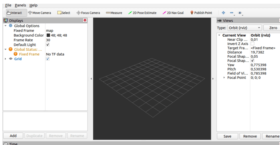
Slika 13. RViz [15]
