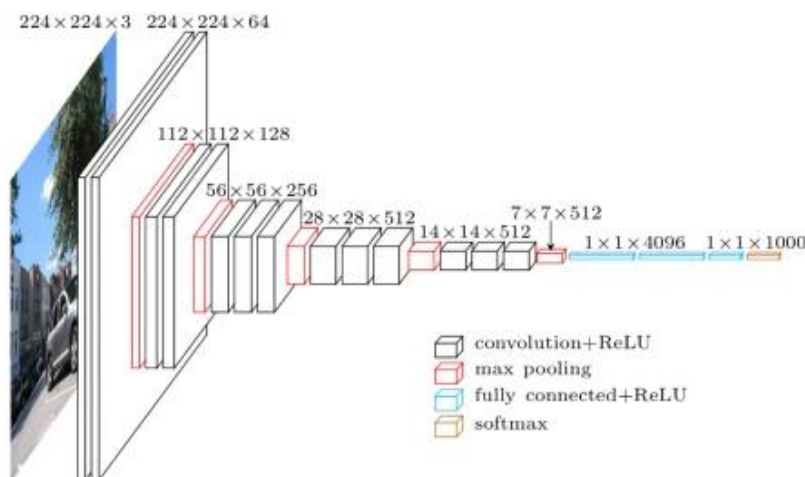
Slika 7. Arhitektura VGG neuronske mreže
