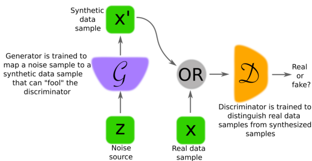
Slika 8. GAN proces [10]
