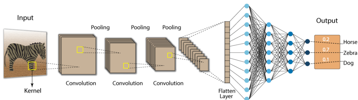
Slika 4. CNN proces [15]
