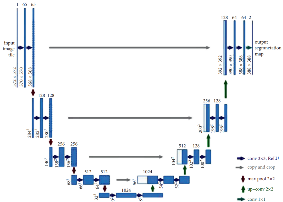
Slika 7. U-Net proces [9]
