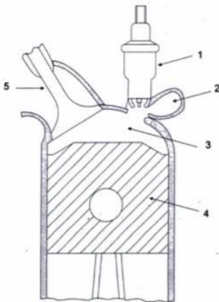
Slika 2. Glavni prostor izgaranja i TGP [6], 1-svjećica, 2-TGP, 3-glavni prostor izgaranja, 4-klip, 5-usisni ventil
