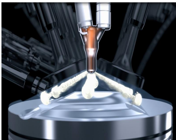
Slika 7. Aktivna pretkomora tvrtke MAHLE Powertrain [10]
