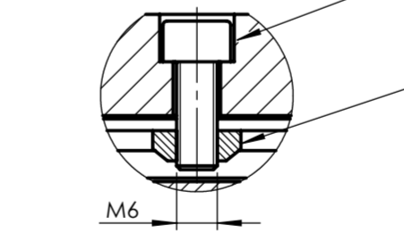
detalj J (M1:1)
