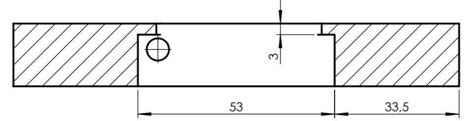
presjek C-C
