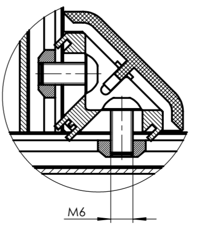
detalj M (M1:1)
