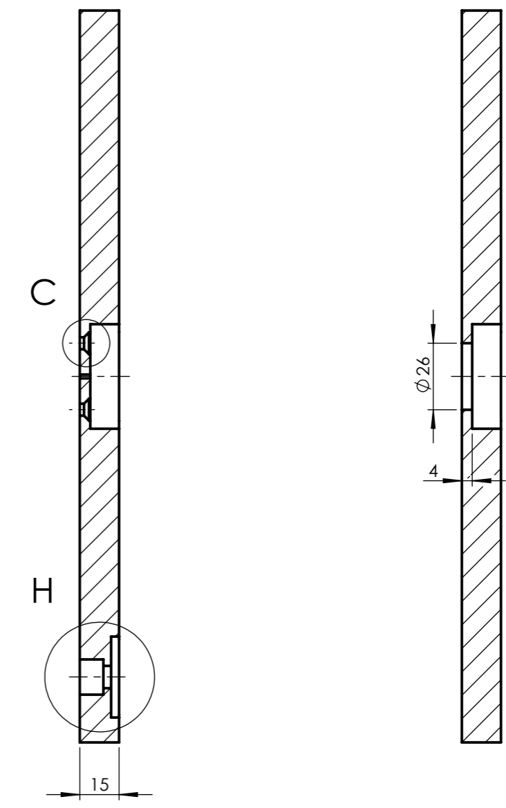
presjek A-A
