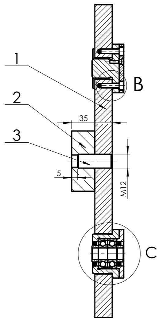
presjek A-A
