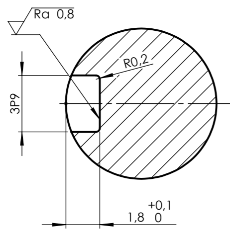
presjek A-A
