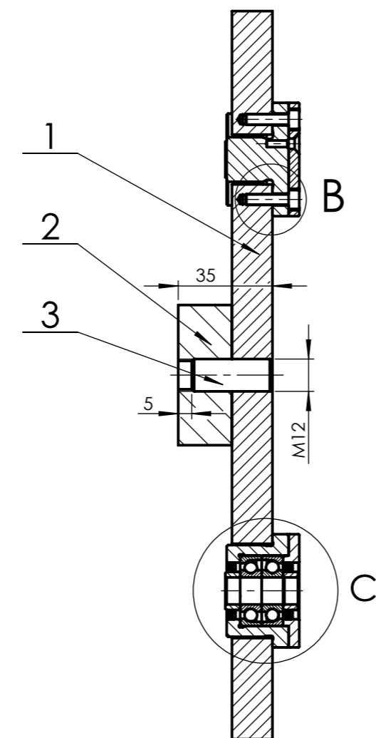
presjek A-A
