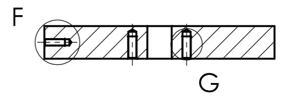
presjek B-B
