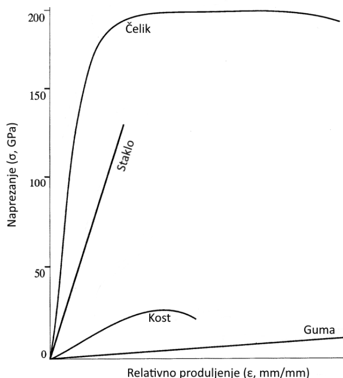
Slika 42. Dijagram naprezanja [62]
