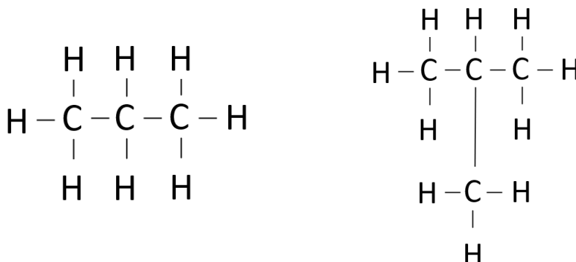
Slika 2. Kemijske strukture propana i izo-butana
