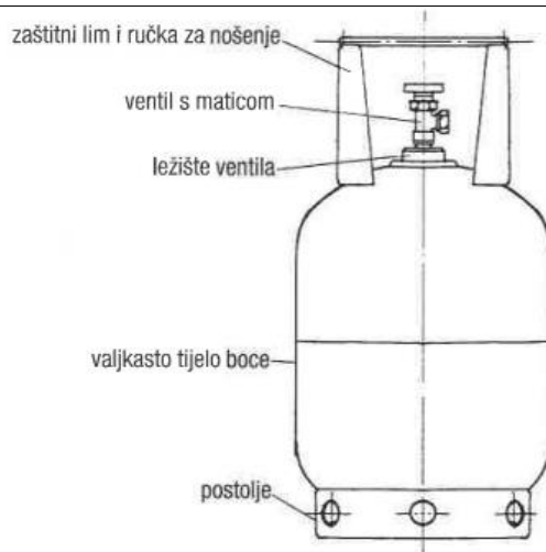
Slika 13. Osnovni dijelovi plinske boce mase 10 kg [9]
