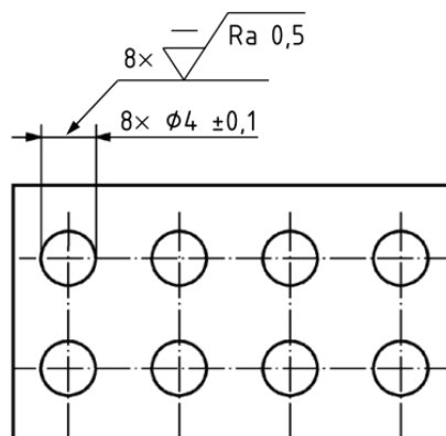
Slika 3.13 Oznaka istih specifikacija za nekoliko istih elemenata [2]
