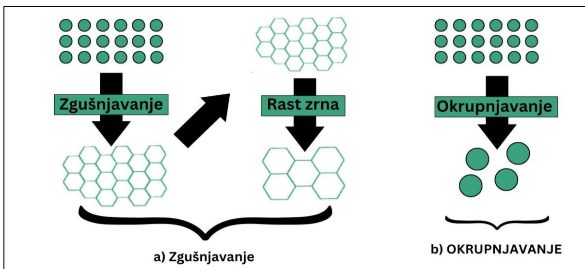
Slika 12. Shematski prikaz (a) zgušnjavanja i (b) okrupnjavanja [13].
