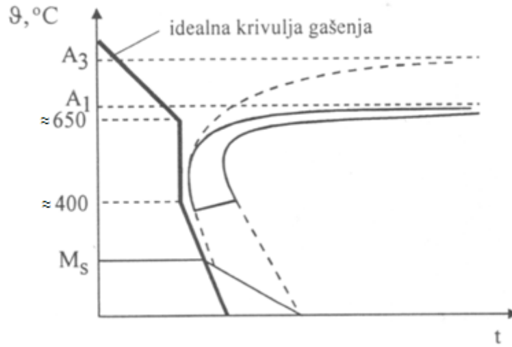
Slika 7. "Idealizirana" krivulja gašenja u TTT dijagramu za kontinuirano ohlađivanje nekog podeutektidnog ugljičnog čelika [6]
