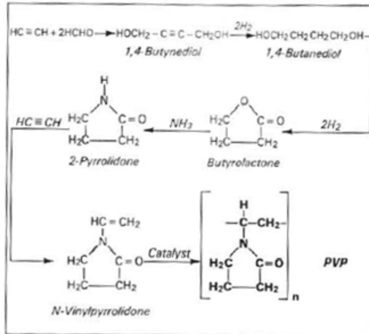
Slika 32. Šest koraka sinteze polimera PVP [18]
