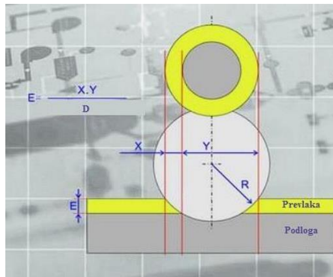
Slika 24. Mjerenje debljine prevlake kalotestom [26]
