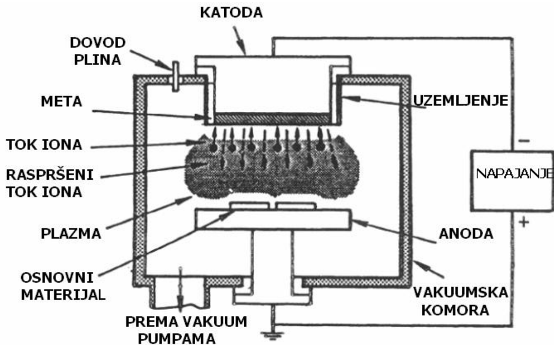
Slika 19: Shematski prikaz PVD postupka aspršivanja materijala prevlake planarnom diodom [2]
