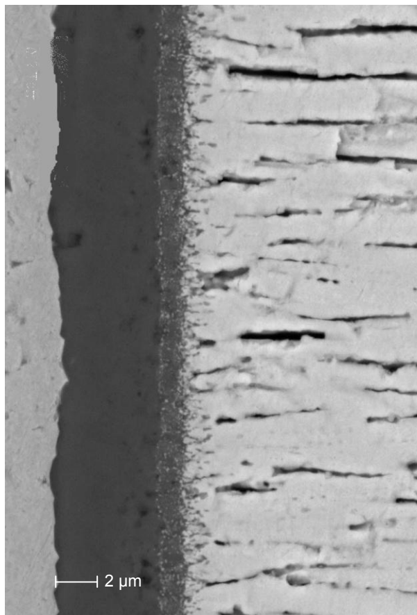
Slika 70: Sastav TBC prevlake na bazi cirkonijeva dioksida [34]
