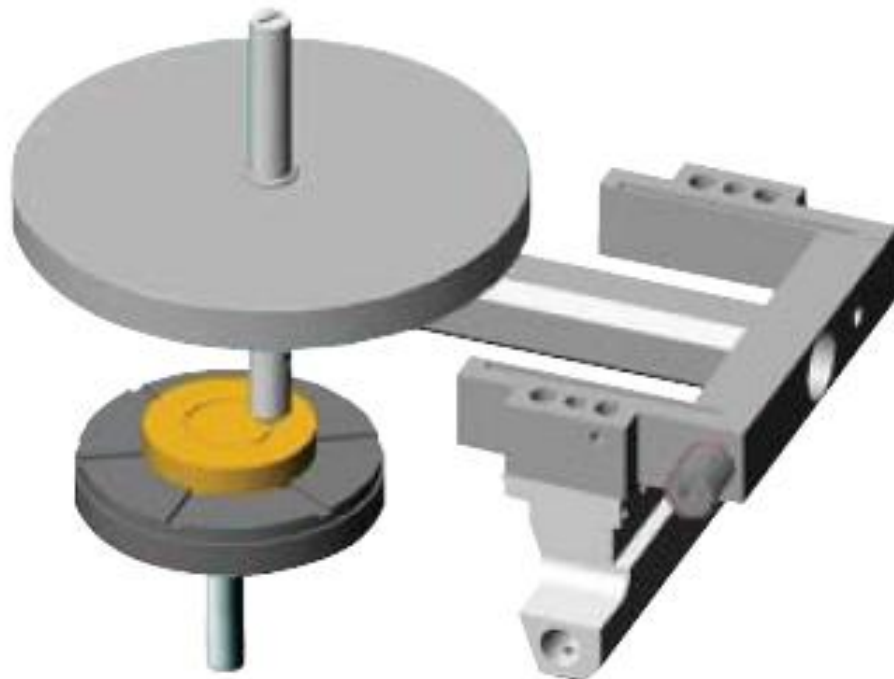
Slika 57: Shematski prikaz ispitivanja triboloških svojstava prevlaka metodom pin-on-disc [22]
