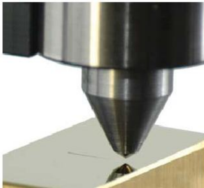
Slika 53: Glava modernog uređaja sa penetratorom za ispitivanje adhezije prevlake na supstrat brazdanjem [22]
