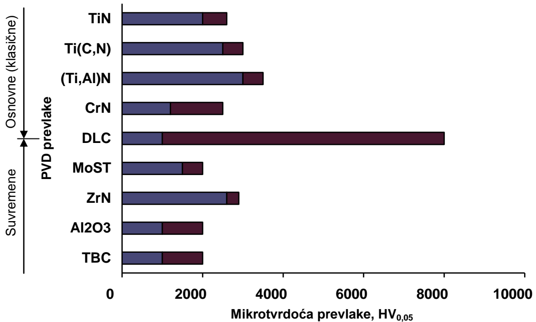
Slika 74: Raspon iznosa mikrotvrdoće PVD prevlaka
