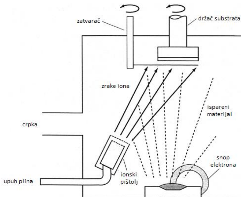
Slika 32: Shematski prikaz sustava za vakuurno ionsko platiniranje [3]
