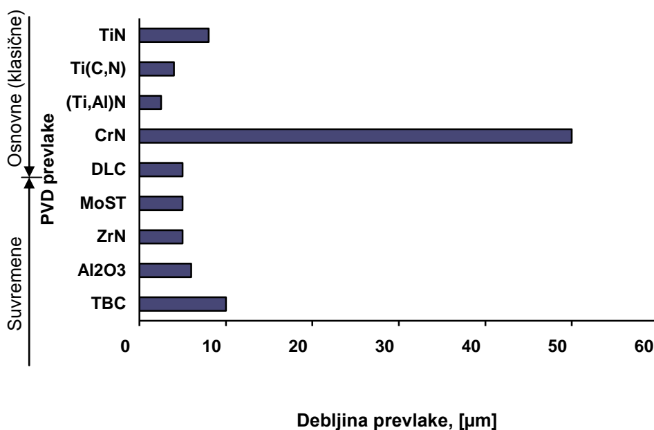
Slika 72: Usporedba debljina PVD prevlaka
