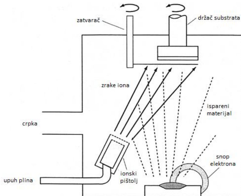
Slika 32: Shematski prikaz sustava za vakuumno ionsko platiniranje [3]
