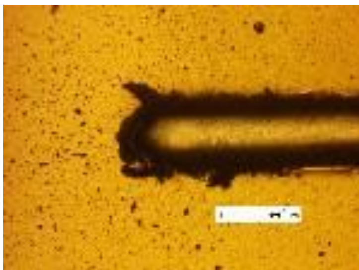
Slika 52: Izgrebeni kanal nakon ispitivanja brazdanjem na prevlaci TiN dobivenoj PVD postupkom s magnetskim raspršivanjem materijala prevlake [8]
