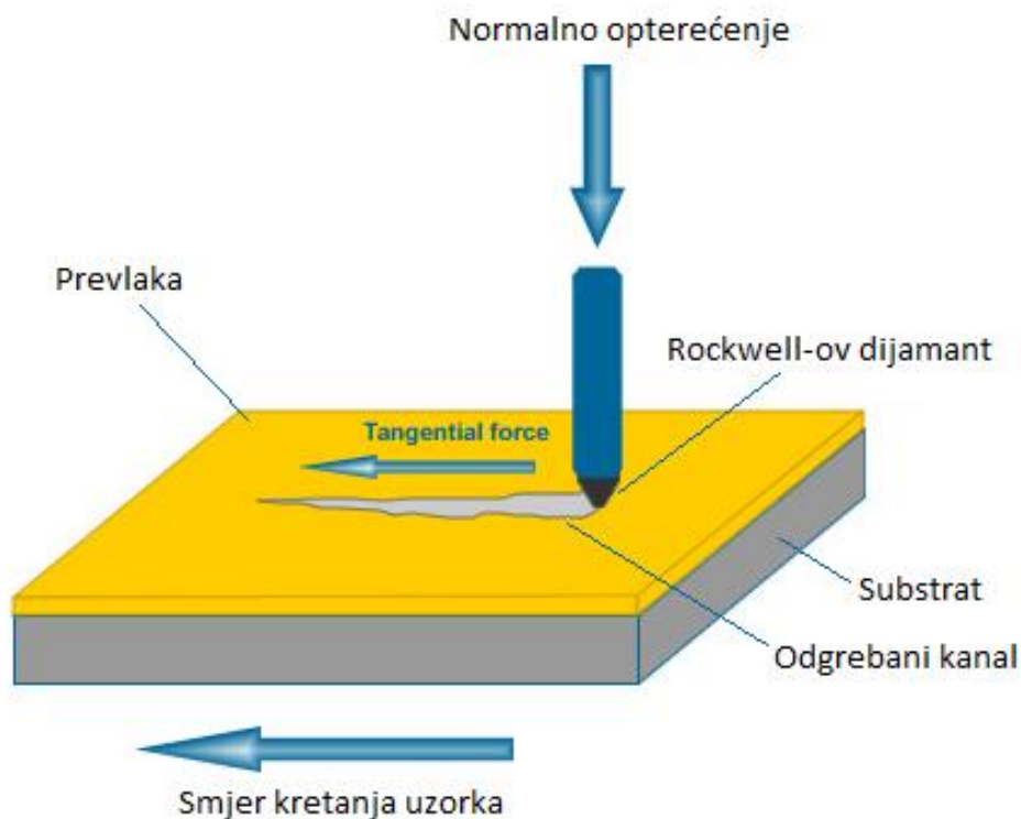
Slika 50: Princip ispitivanja adhezije prevlake na substrat brazdanjem [8]
