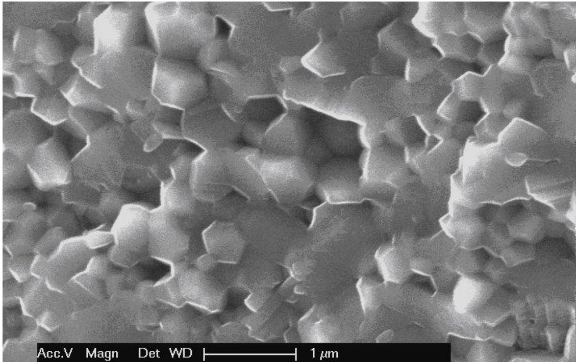
Slika 42: Mikroskopska snimka PVD prevlake \text{Al}_2\text{O}_3 [16]
