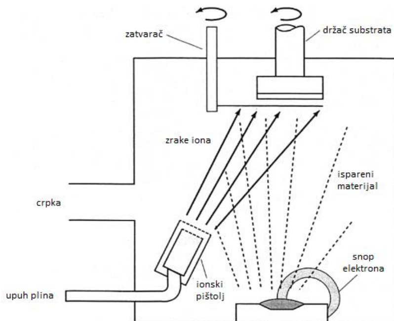
Slika 32: Shematski prikaz sustava za vakuumske ionske platiniranje [3]
