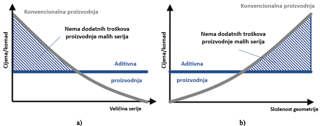
Slika 4. Usporedba: a) ovisnost cijene o veličini serije; b) ovisnost cijene od složenosti geometrije za aditivnu proizvodnju i konvencionalni način proizvodnje [65]
