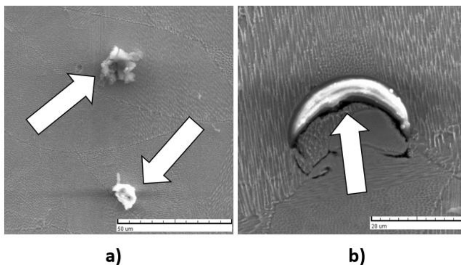
Slika 40. Primjer neželjenih uključina bogatih silicijem u mikrostrukтури ispitnog uzorka: a) 5-4-Z, b) 3-2-Z, SEM
