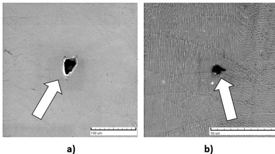
Slika 39. Porozitet u mikrostrukтури ispitnog uzorka: a) 15-3-Z, b) 5-4-Z, SEM
