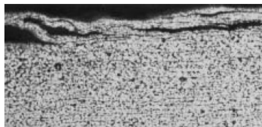
Greške na unutrašnjoj površini zbog nečistoća u čeliku
