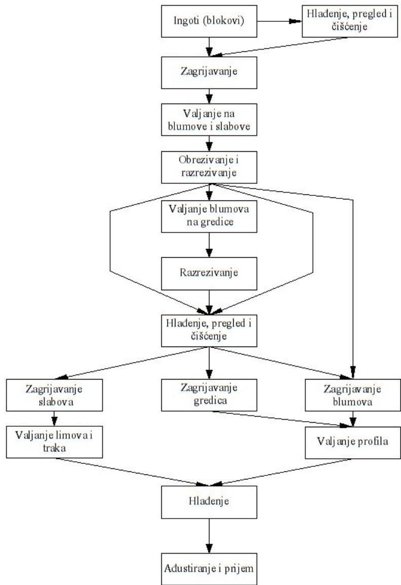
Slika 1.3 Shema valjaoničke proizvodnje [1]
