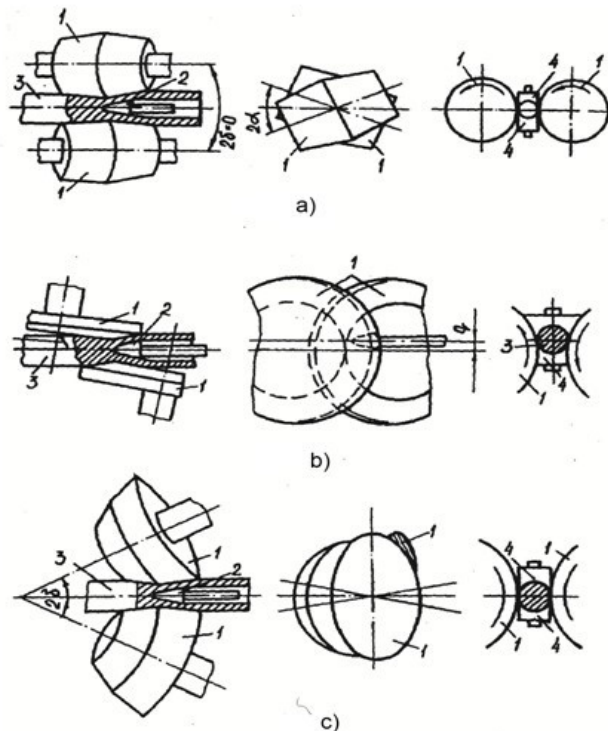
Slika 3.2. Sheme bušućih stanova s oblikom valjaka: bačvastim (a), i diskovima (b), i gljivastim (c) (1 – valjak, 2 – trn, 3 – uložak – cijevnica, 4 – vodilice matrice) [1]
