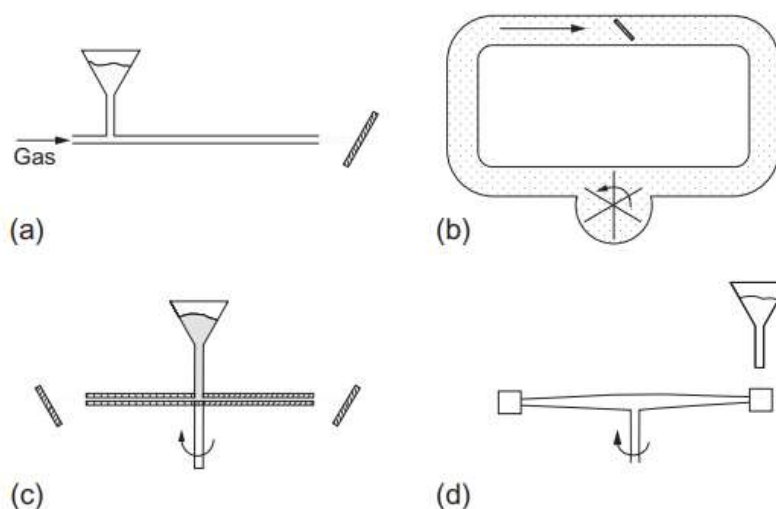
Slika 18. Prikaz eksperimentalnih metoda određivanja otpornosti na trošenje erozijom [4]
