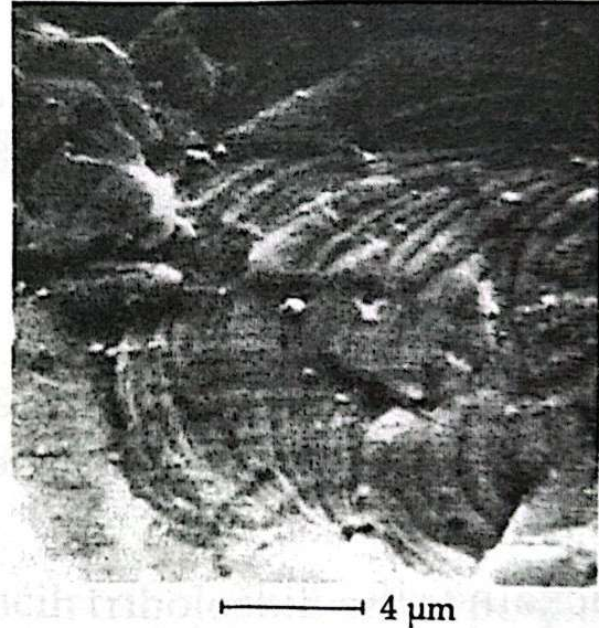
Slika 9. Površina oštećena umorom [4]
