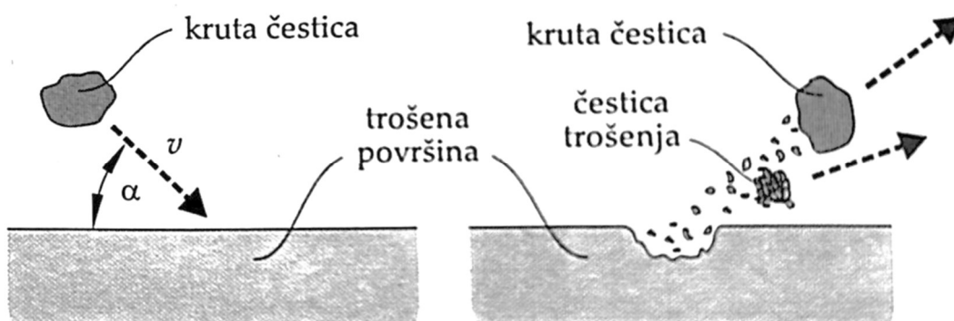
Slika 12. Prikaz upada erozijske čestice i odošenja čestice materijala [5]
