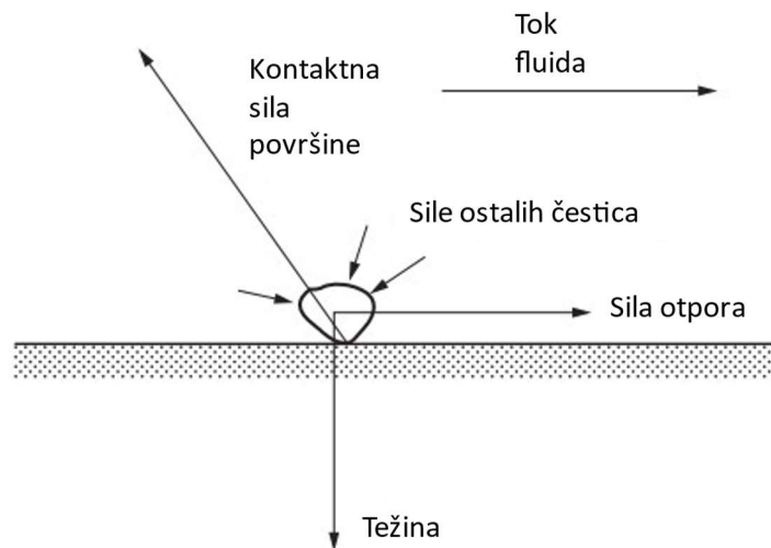
Slika 11. Inicijalni događaj erozije [4]
