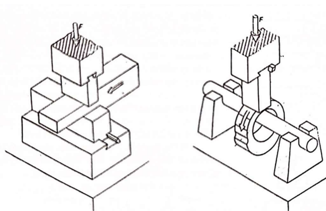
Slika 22. Postupak iskivanja [6]
