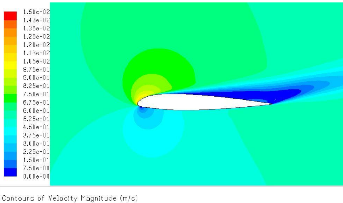
Slika 5.8: Raspored brzine oko aeroprofila s naslagom leda pri 15°
