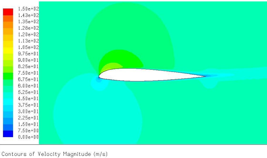
Slika 5.7: Raspored brzine oko aeroprofila s naslagom leda pri 5°
