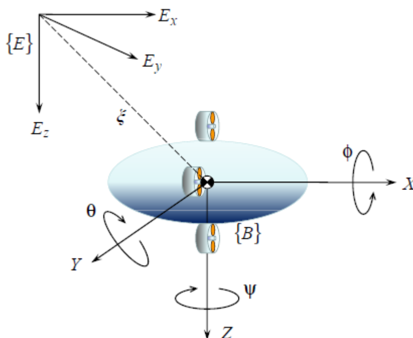
Slika 3.2 Koordinatni sustavi [1]
