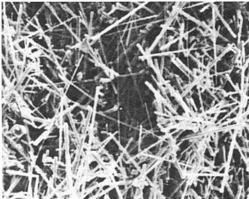
Slika 20. Prikaz SiC whiskera pod povećanjem od 1250 \times [4]
