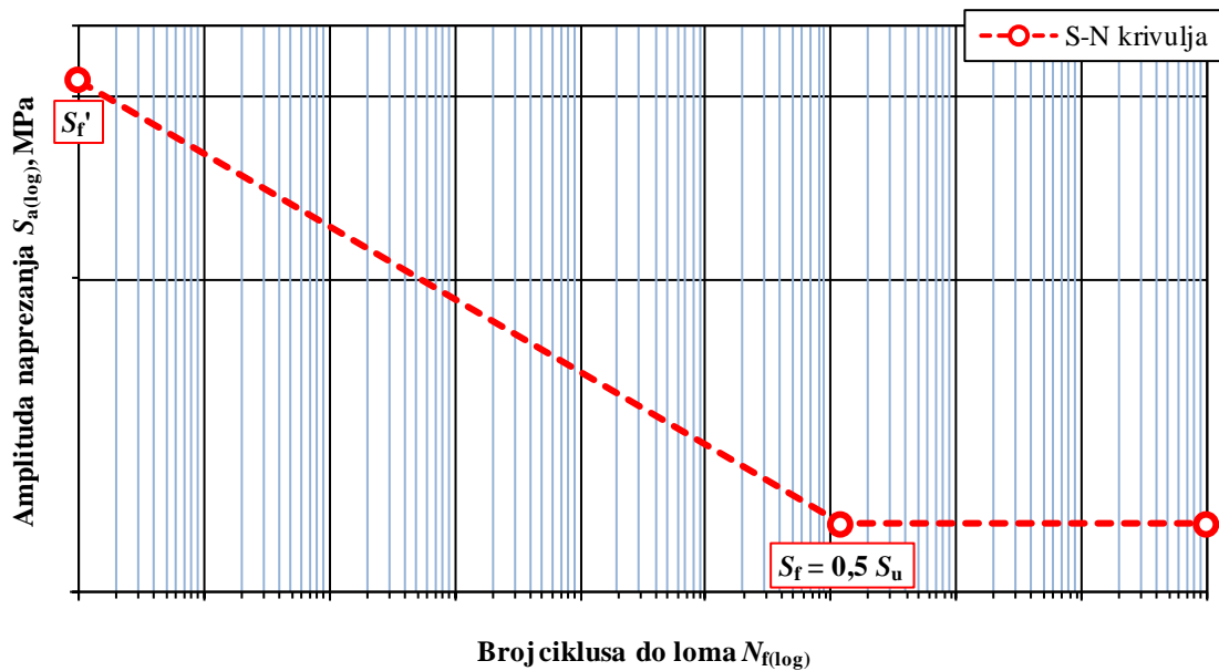
Slika 4. S - N metoda [2]
