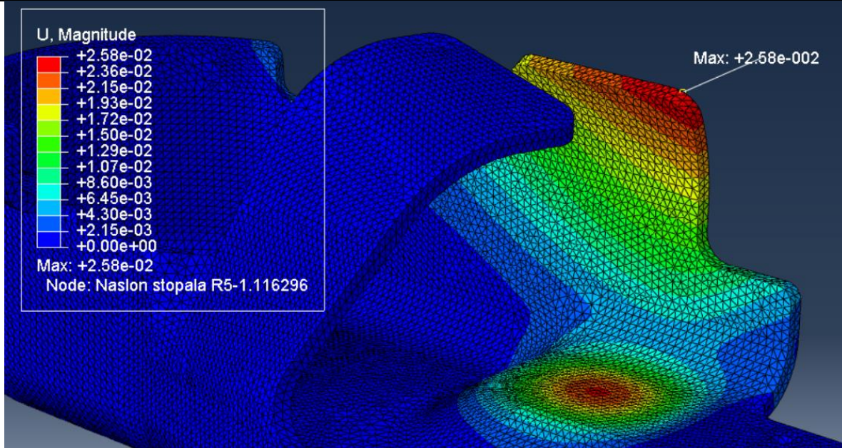
Slika 80. Prikaz maksimalnih pomaka naslona za stopalo
