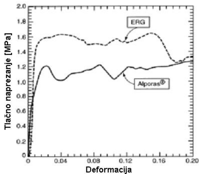
Slika 5.4. Dijagram naprežanje-deformacija otvorenih (ERG) i zatvorenih (Alporas) metalnih pjena. [3]
