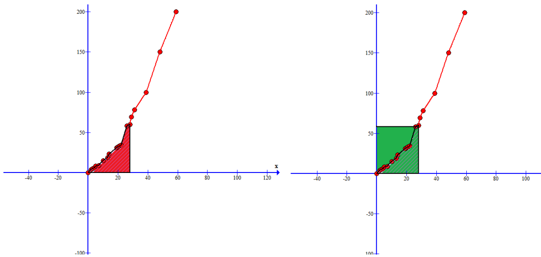
Slika 5.11. Apсорbirana deformacijska energija (lijevo, crvena) i energija idealnog apsorpcijskog materijala (desno, zeleno)
