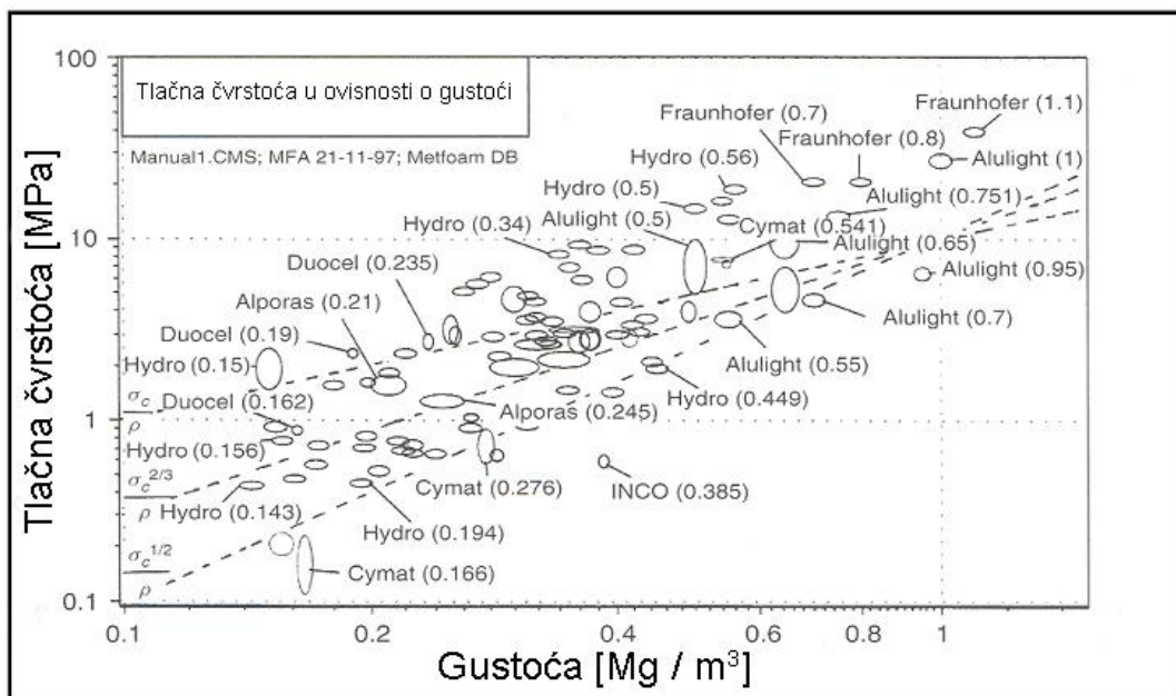
Slika 5.6. Prikaz vrijednosti tlačne čvrstoće u ovisnosti o gustoći za komercijalne metalne pjene. [4]
