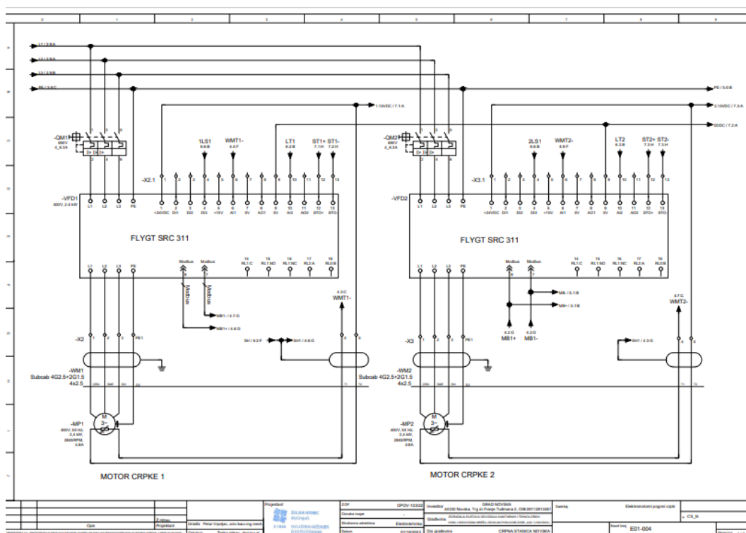
Slika 9: Shema upravljačkog ormarića – Stranica 4
