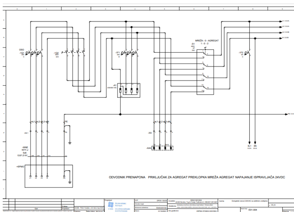
Slika 6: Shema upravljačkog ormarića – Stranica 1
