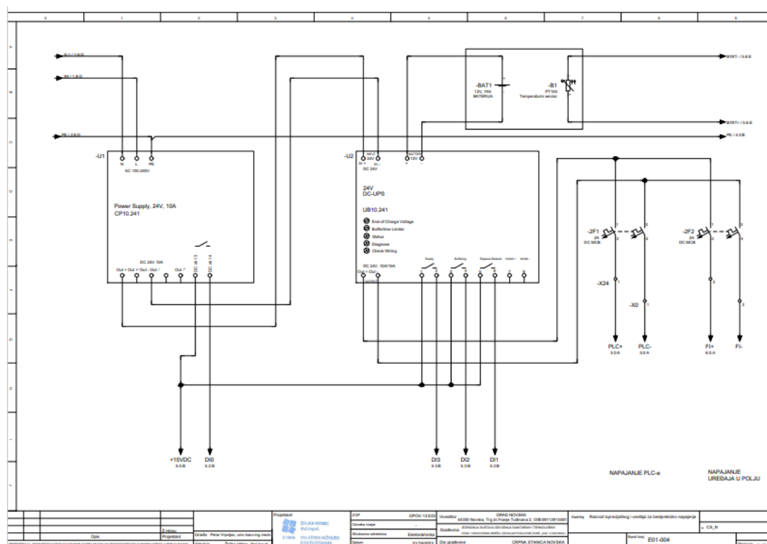
Slika 8: Shema upravljačkog ormarića – Stranica 3
