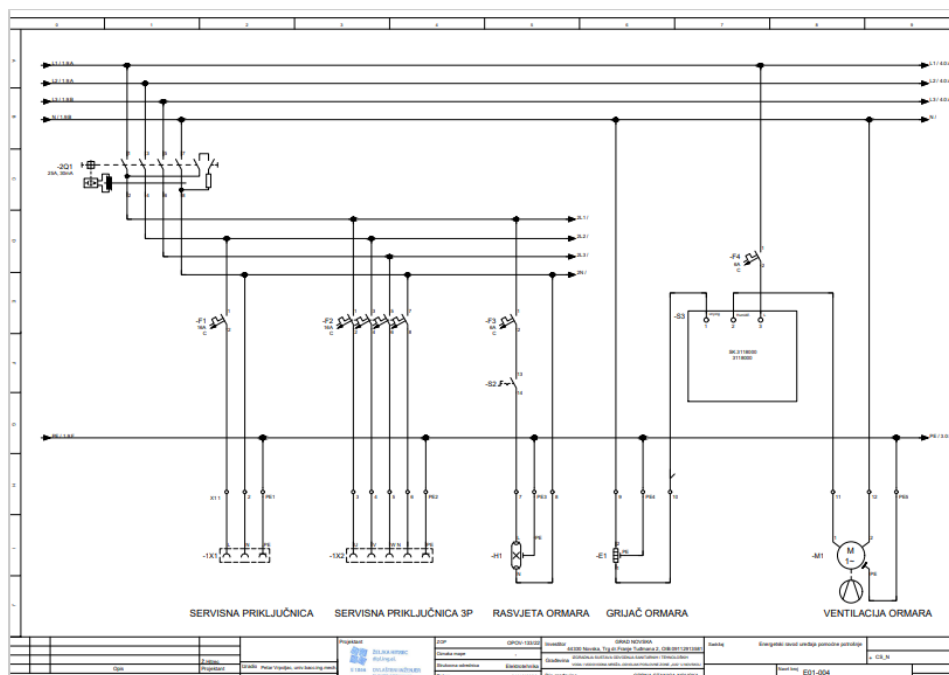
Slika 7: Shema upravljačkog ormara – Stranica 2
