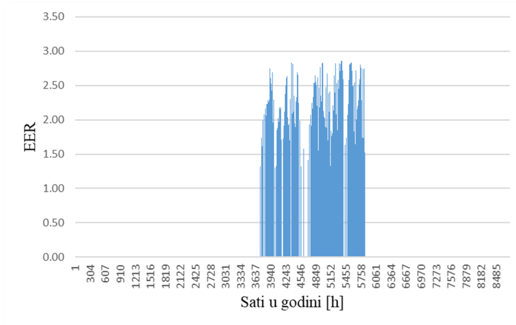
Slika 23 Vrijednosti EER-a dizalice topline u režimu hlađenja
