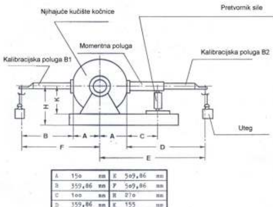
Slika 8.1. Razmjštaj i mjere kalibracijske poluge
