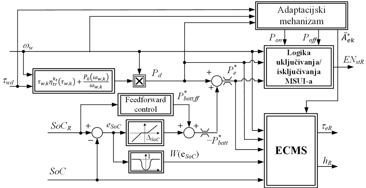
Slika 6-1. Blokovski dijagram adaptivne RB+ECMS-EXT strategije upravljanja PHEV-om.
